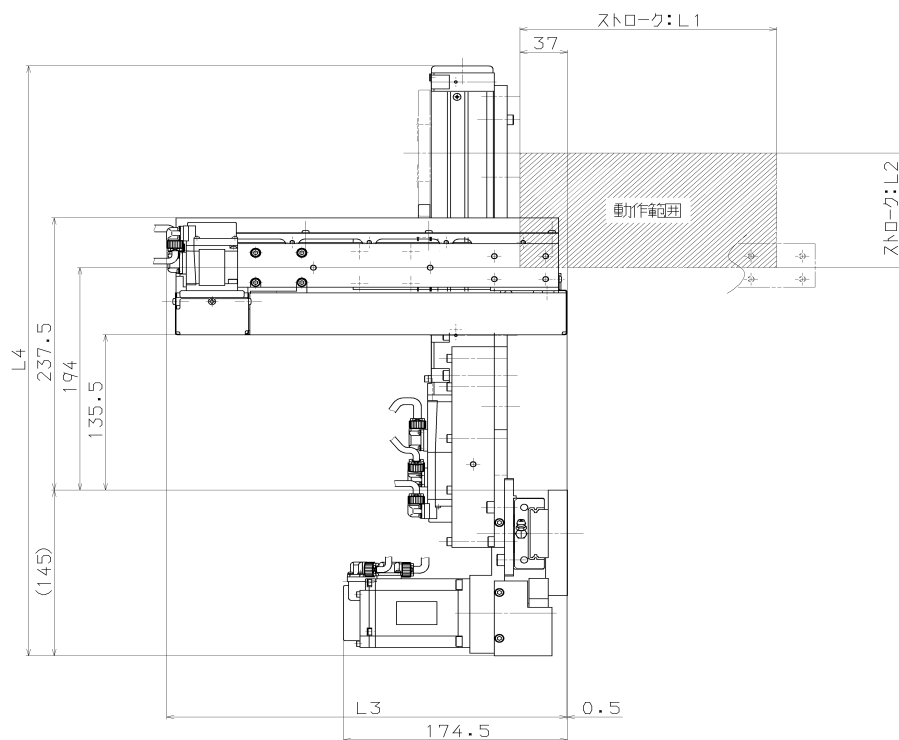
S轴头的安装尺寸
