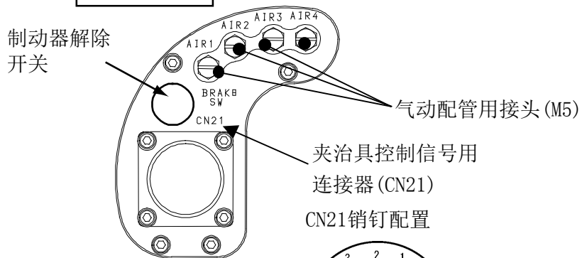
(A) 箭头视图
