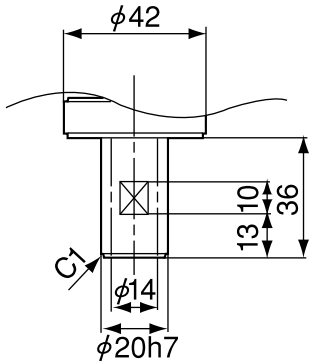
工具安装面详图（视图D）
