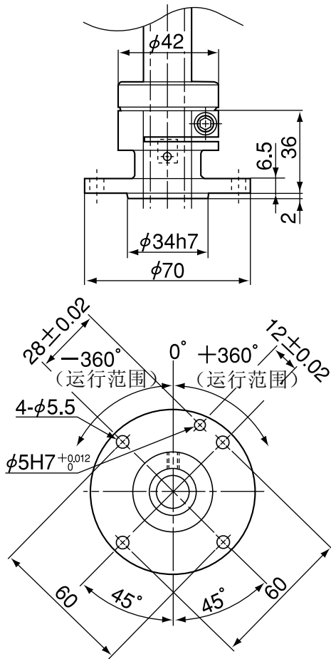
法兰盘（选件）安装图
