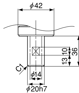
工具安装面详图（箭头视图D）
