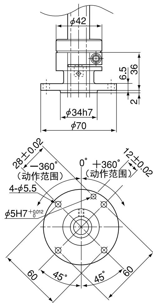
法兰（选件）安装图
