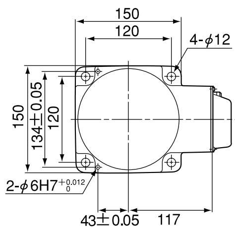
底座安装尺寸
