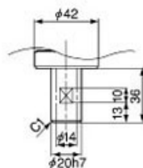
工具安装面详图 (箭头视图 D)
