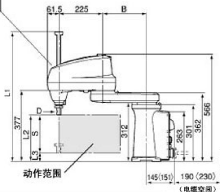
底座安装尺寸
