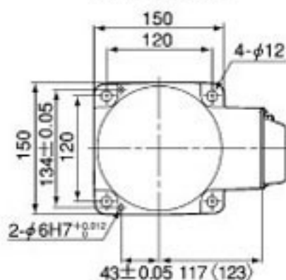
底座安装尺寸
