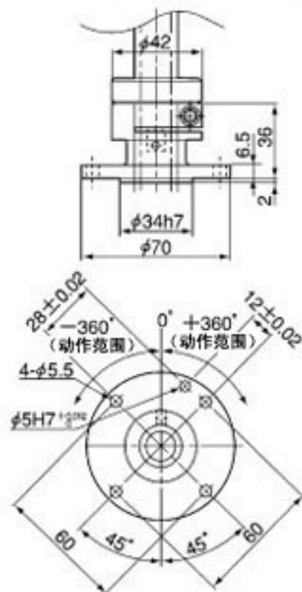
法兰 (选件) 安装图
