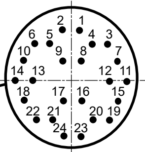
(夹治具控制信号用连接器) CN21销钉排列
