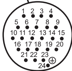
CN20销钉排列 (夹治具控制信号用连接器)
