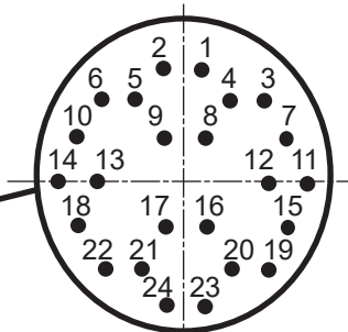
(夹治具控制信号用连接器) CN21销钉排列
