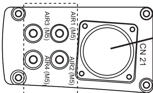
A箭头视图
