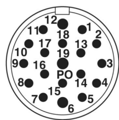
CN20 销钉排列
