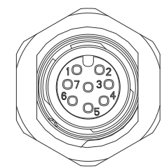
Ethernet连接器销钉排列
