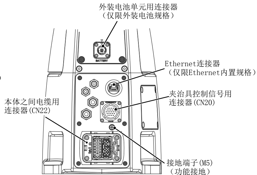
(B) 视图
