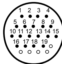
CN20销钉排列
