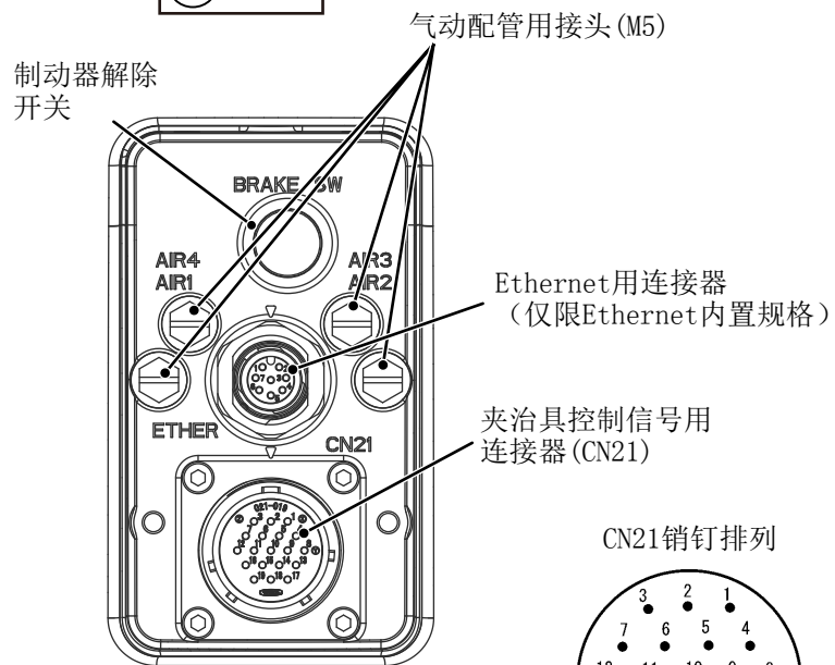
(A) 视图
