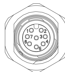
Ethernet连接器销钉排列
