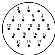
CN21销钉排列
