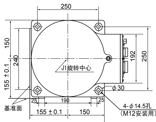
底座安装尺寸（B-B视图）
