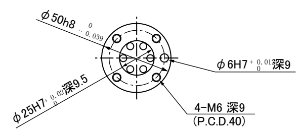
工具安装面详图 (A视图)
