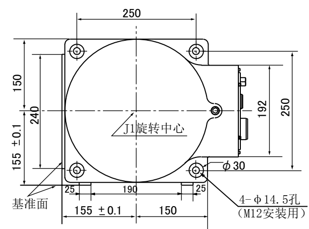
底座安装尺寸 (B-B视图)
