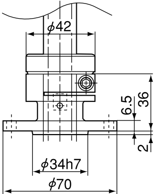
フランジ(オプション)取付図
