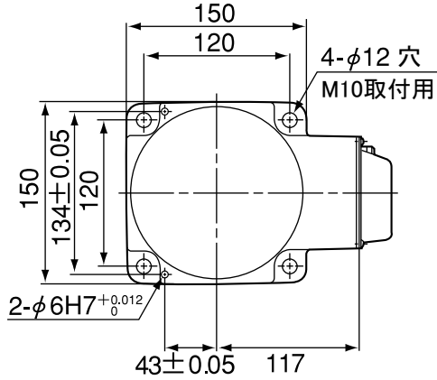
ベース取付寸法
