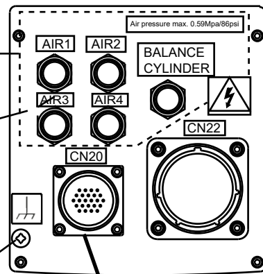
B 矢視図
