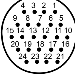
B 矢視図
