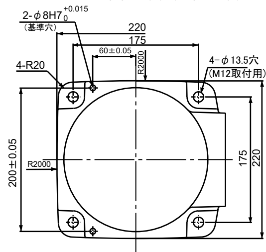
ベース取付寸法 (上面より)
