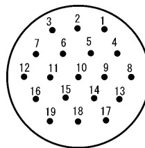
CN21ピン配置
