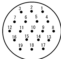
CN21ピン配置
