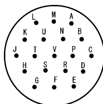
CN20ピン配置
