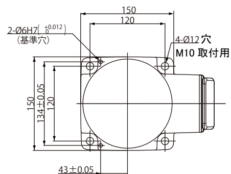
ベース取付寸法
