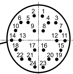
(ハンド制御信号用コネクタ) CN21ピン配置
