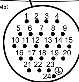
CN20ピン配置 (ハンド制御信号用コネクタ)
