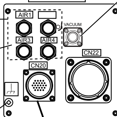
B 矢視図
