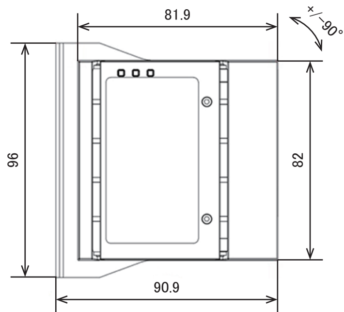
側面
