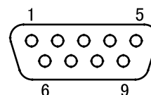
ケーブル側結合面より見た図
