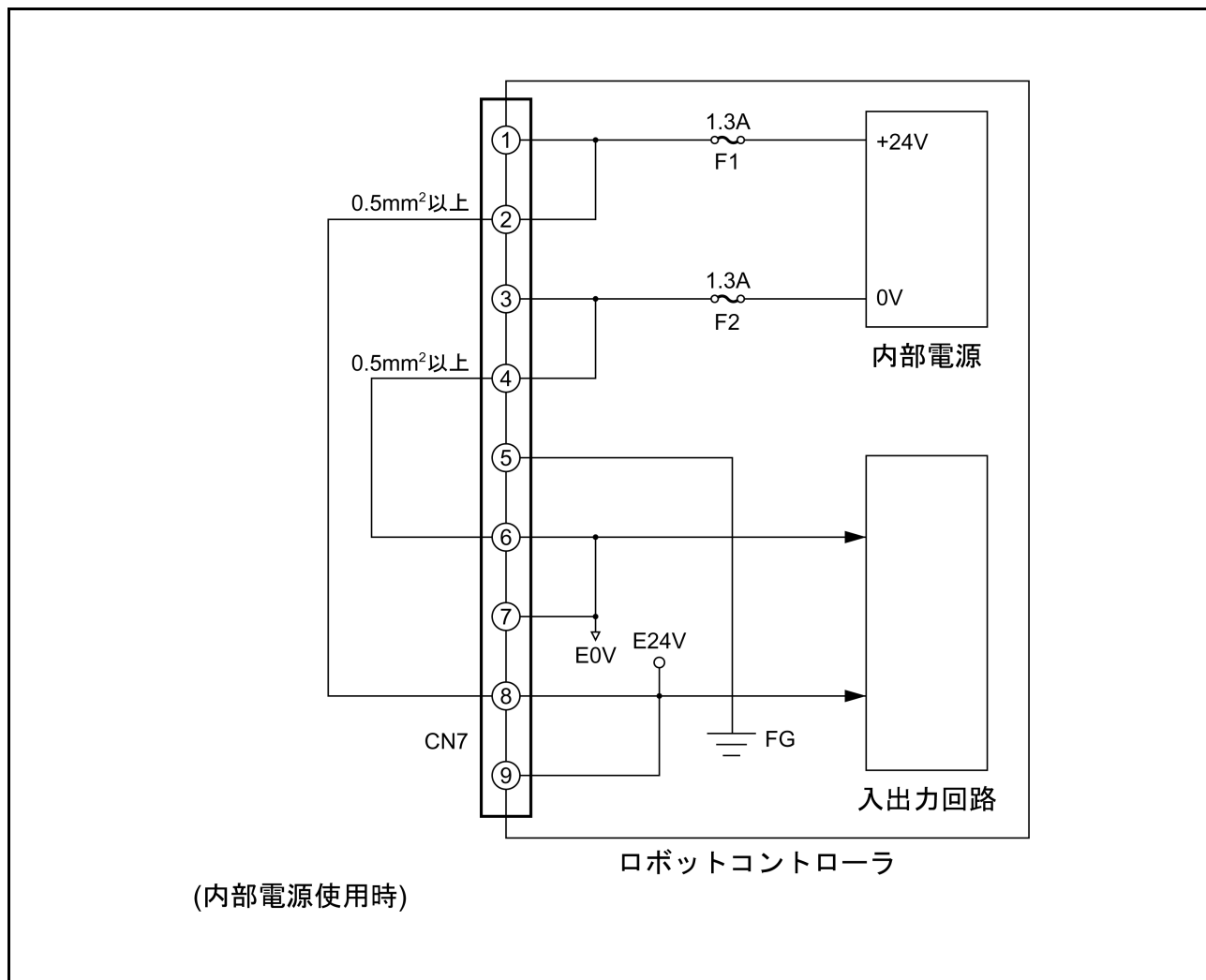
I/Oパワーコネクタ接続例 (PNPタイプI/O)
