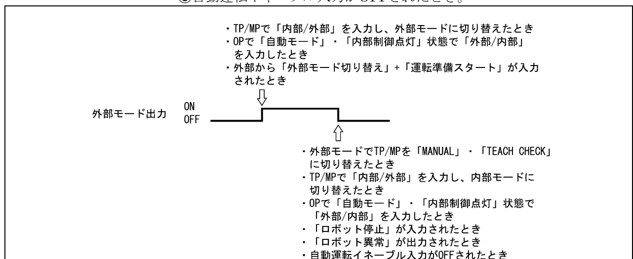
外部モード出力（互換モード）
