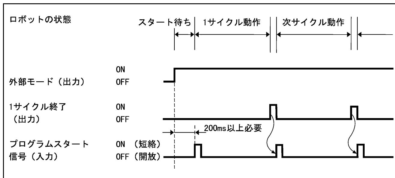
プログラムスタート信号立ち上げのタイミング例（互換モード）
