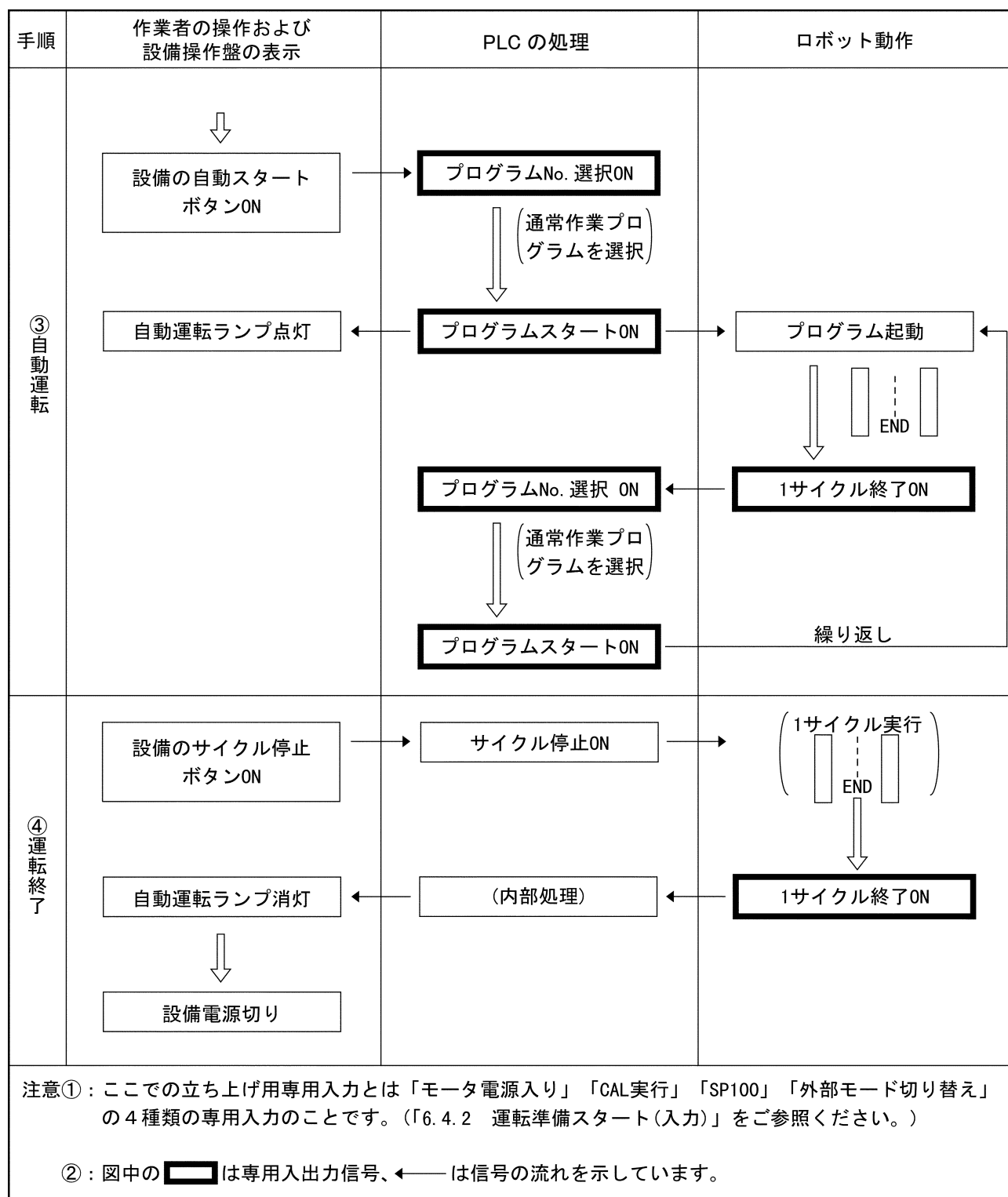
起動・停止の手順と専用入出力信号-2
