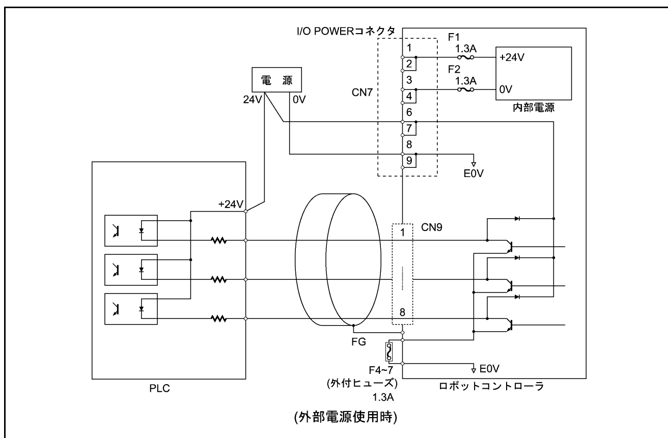
ハンド出力の回路 (NPNタイプI/O)
