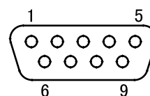
ケーブル側結合面より見た図
