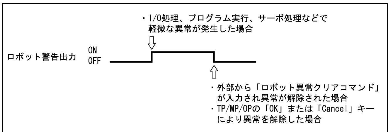
ロボット警告出力（互換モード）
