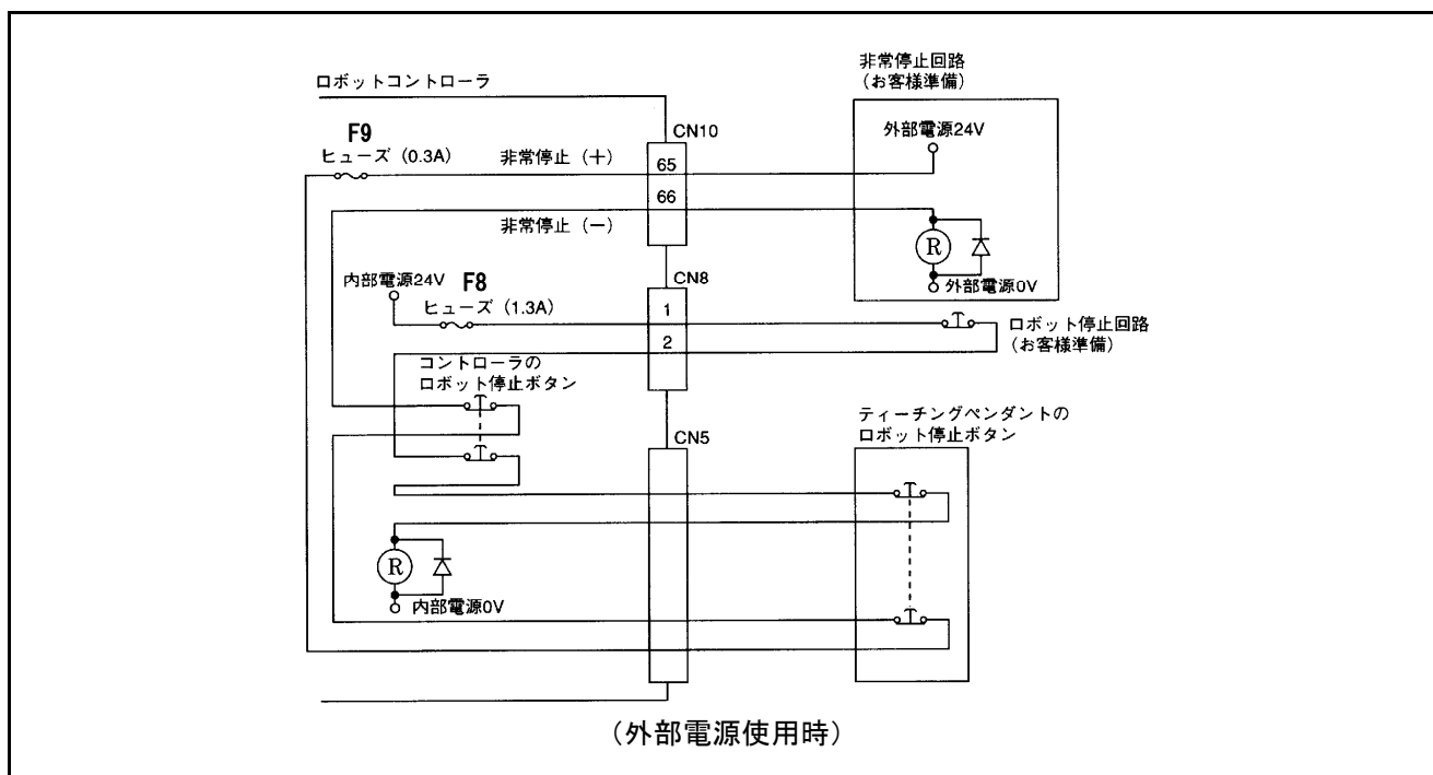
非常停止回路（標準仕様）
