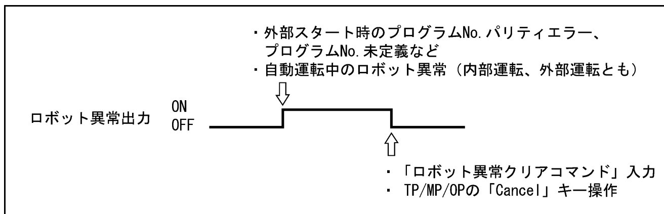
ロボット異常出力（標準モード）
