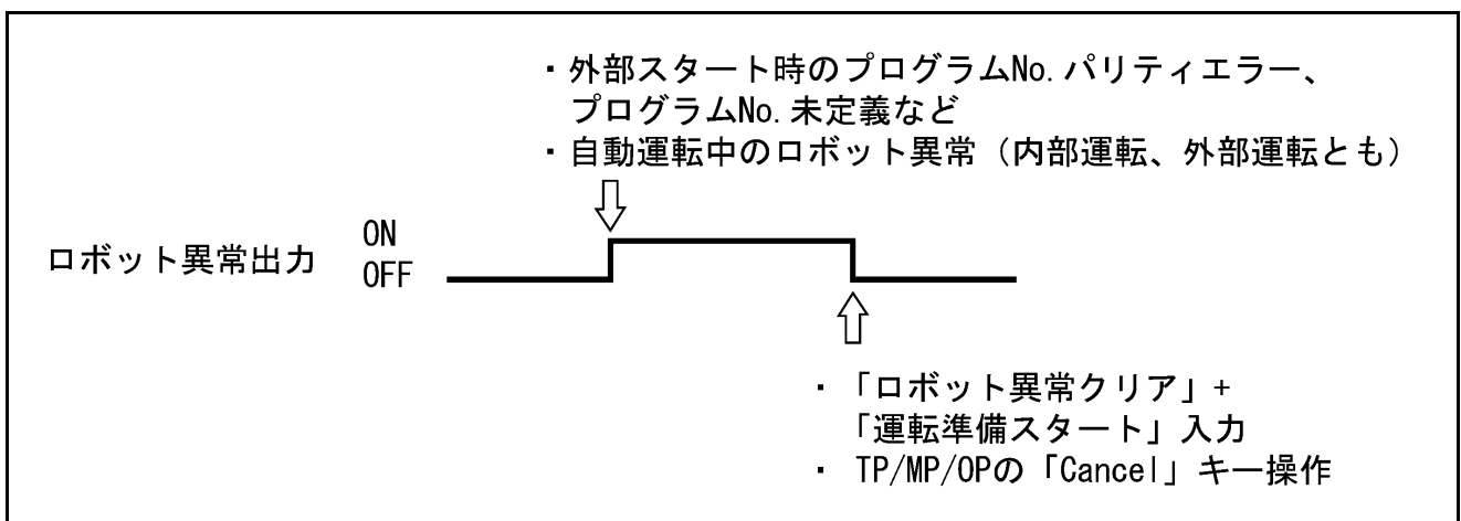
ロボット異常出力（互換モード）
