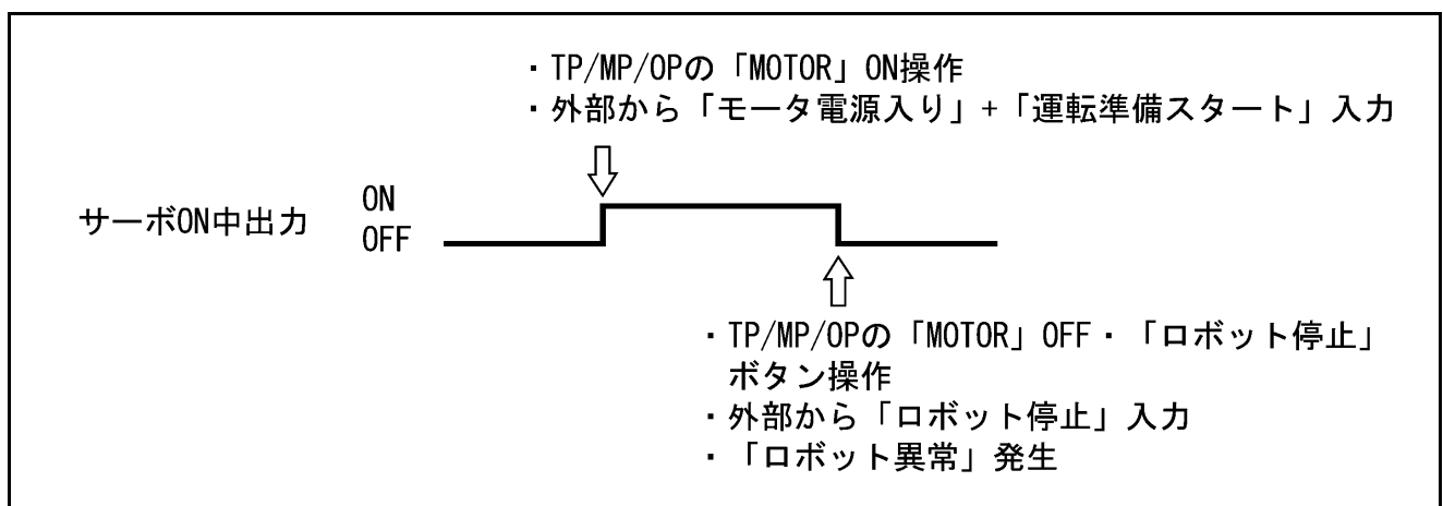
サーボON中出力（互換モード）
