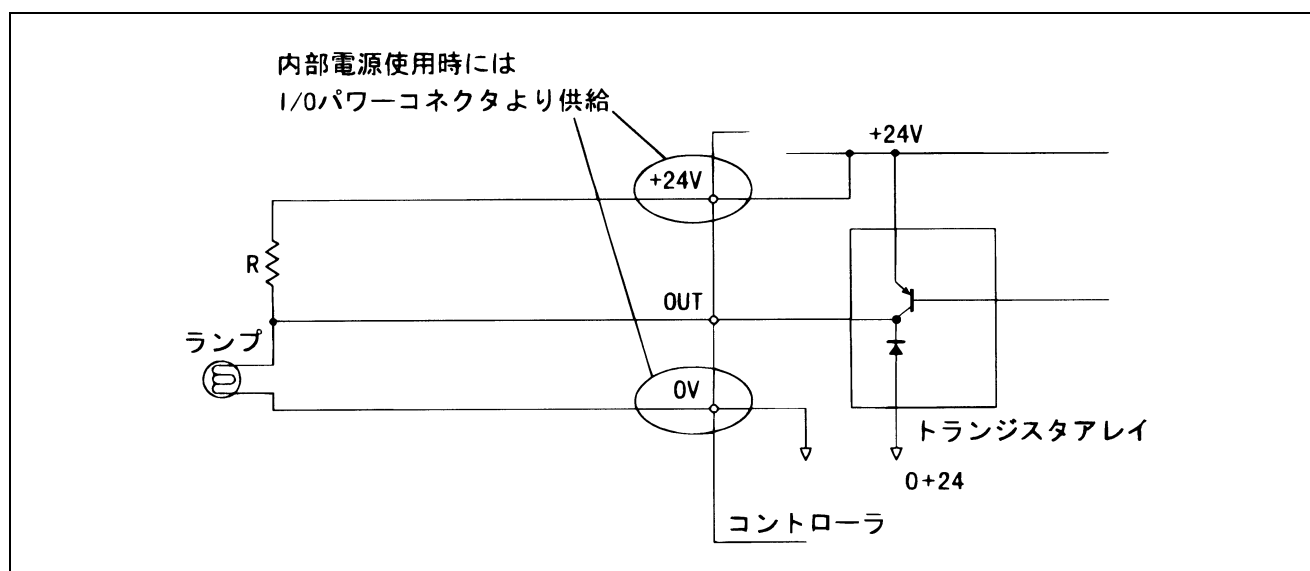
ランプ接続回路例（PNPタイプI/O）
