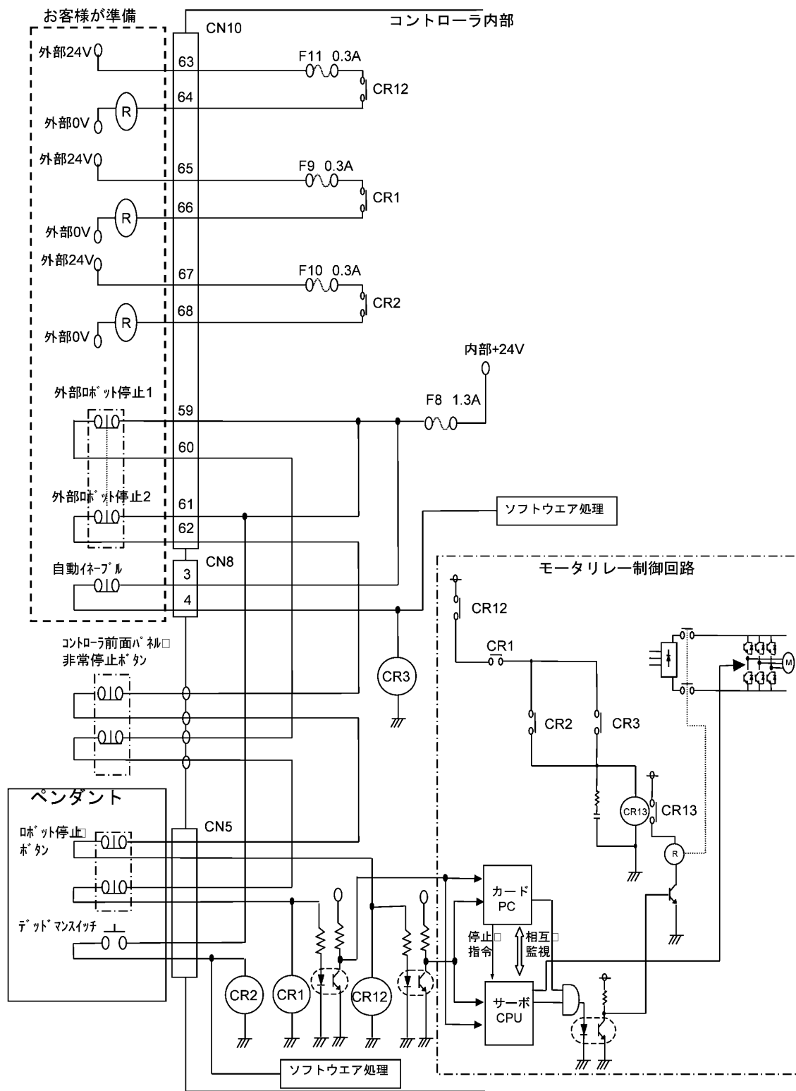
非常停止回路（2重安全仕様）
