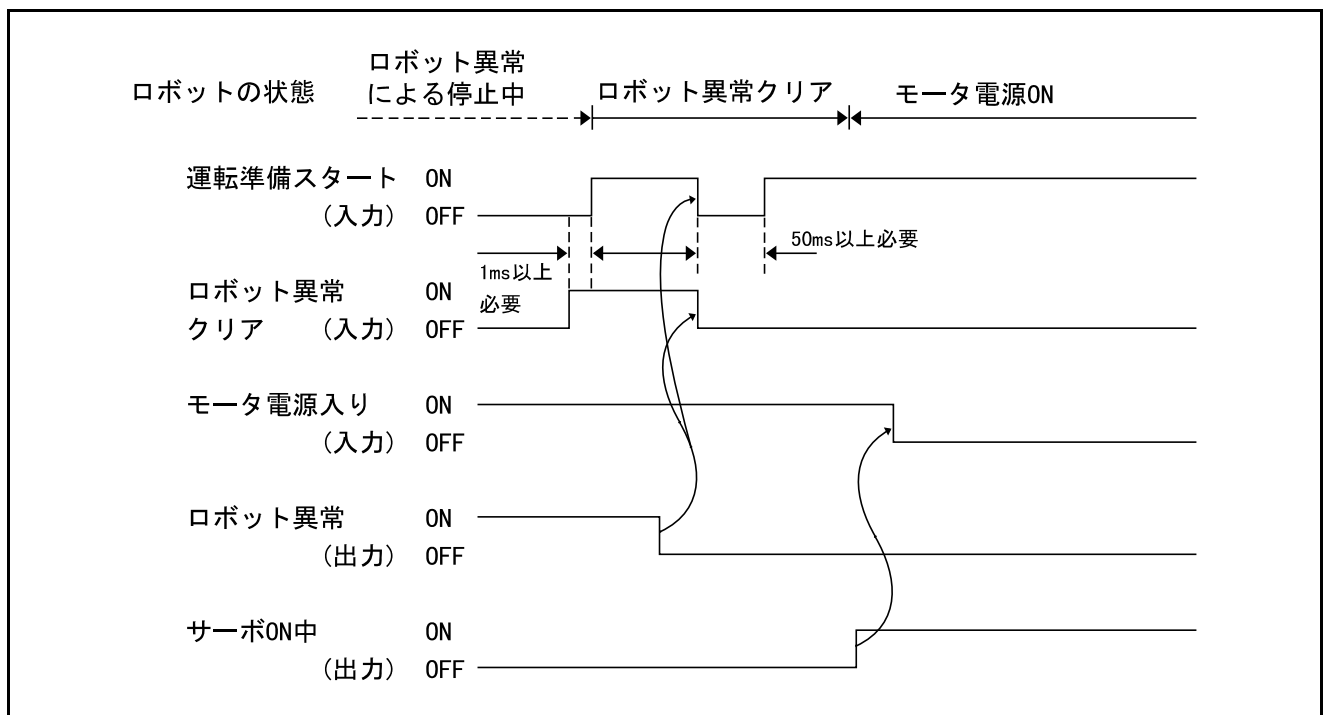
ロボット異常クリア信号の入力条件と動作
