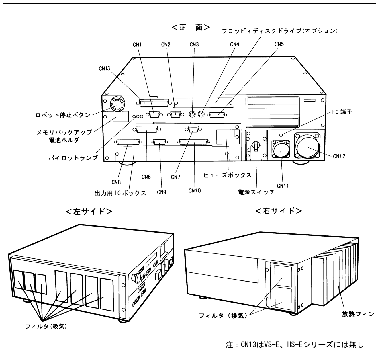
ロボットコントローラ各部の名称 (VM-D/HM-Eシリーズ以外)
