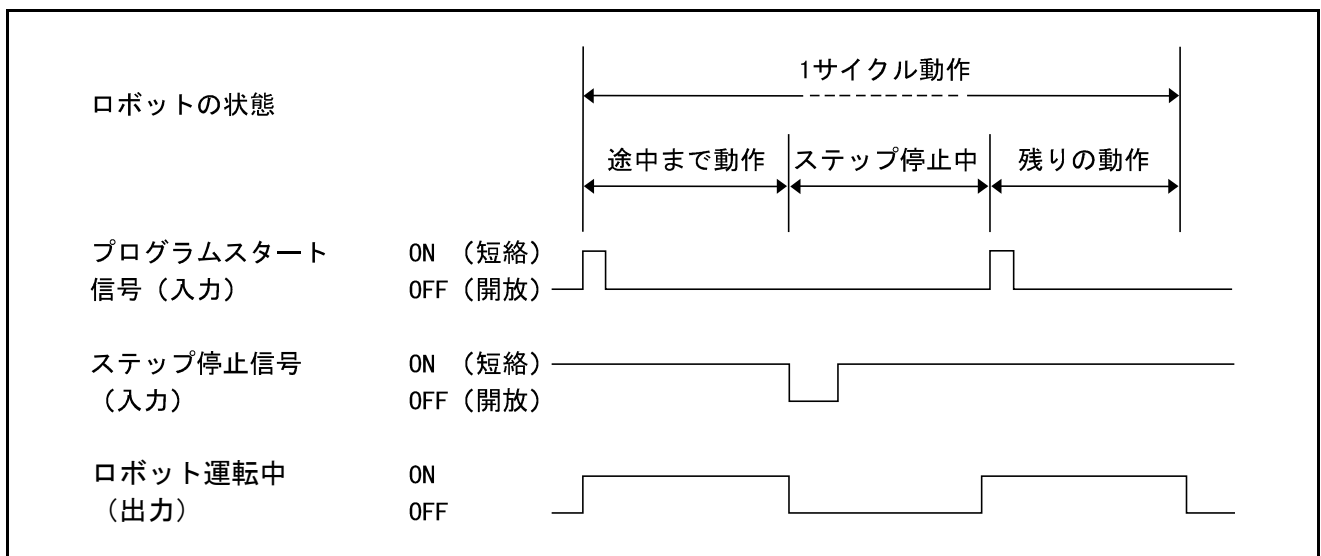
ステップ停止信号
