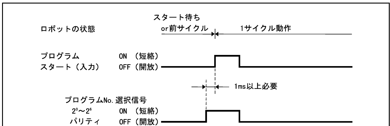
プログラムNo.選択信号（互換モード）
