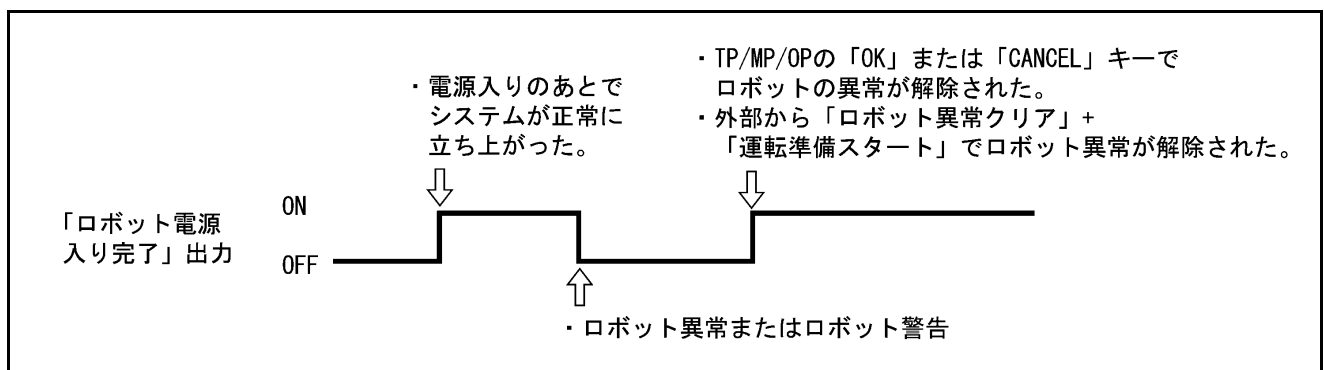
ロボット電源入り完了出力（互換モード）
