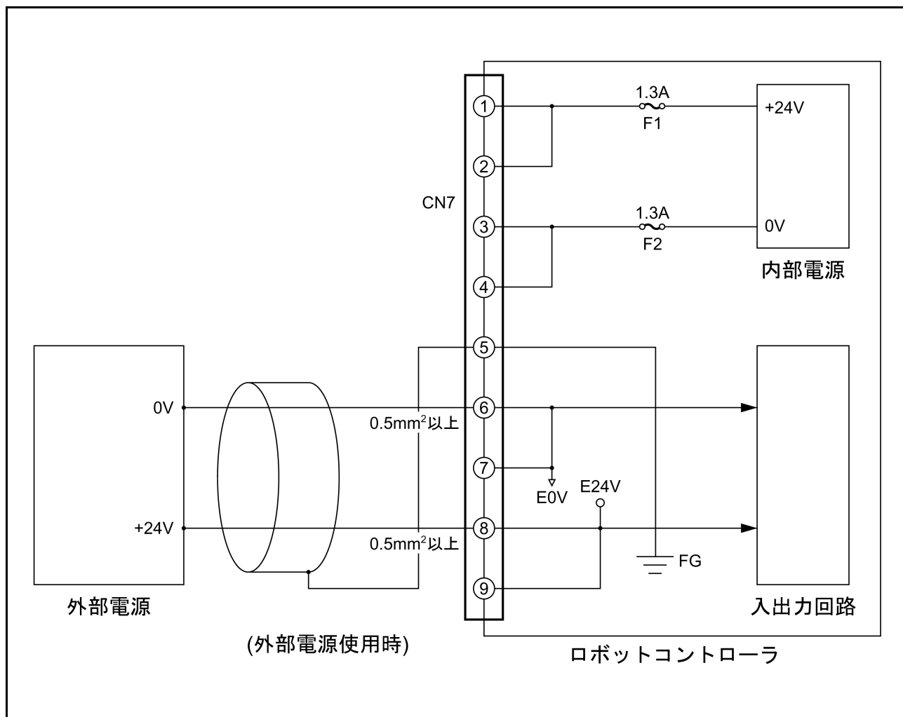
I/Oパワーコネクタ接続例 (PNPタイプI/O)
