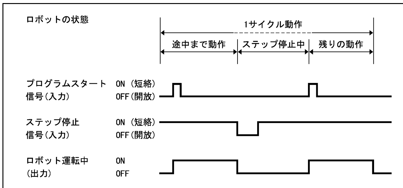
ステップ停止信号（標準モード）
