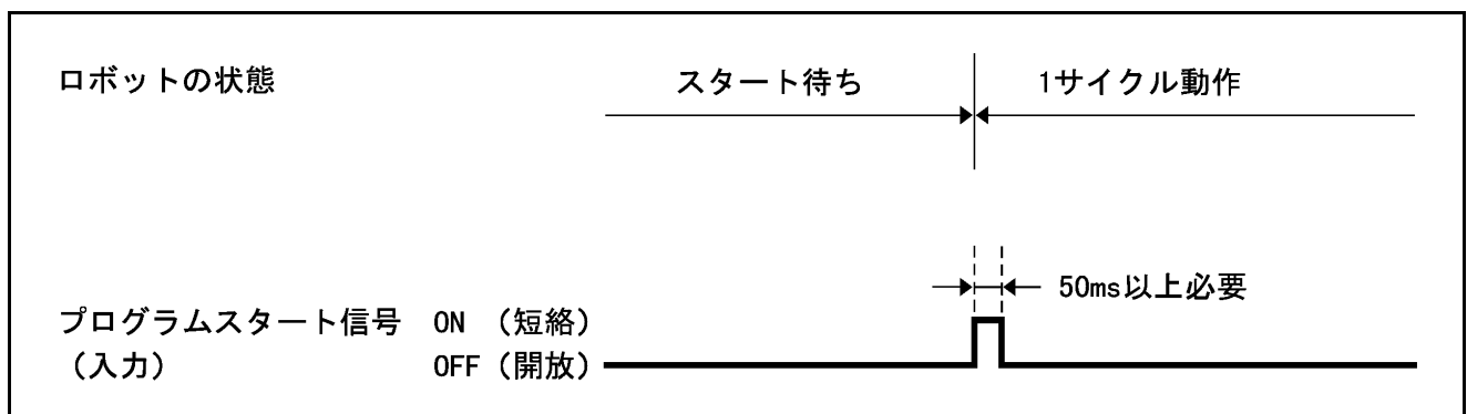
プログラムスタート信号立ち下げのタイミング例 2（互換モード）
