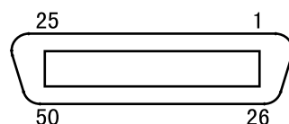
ケーブル側結合面より見た図
