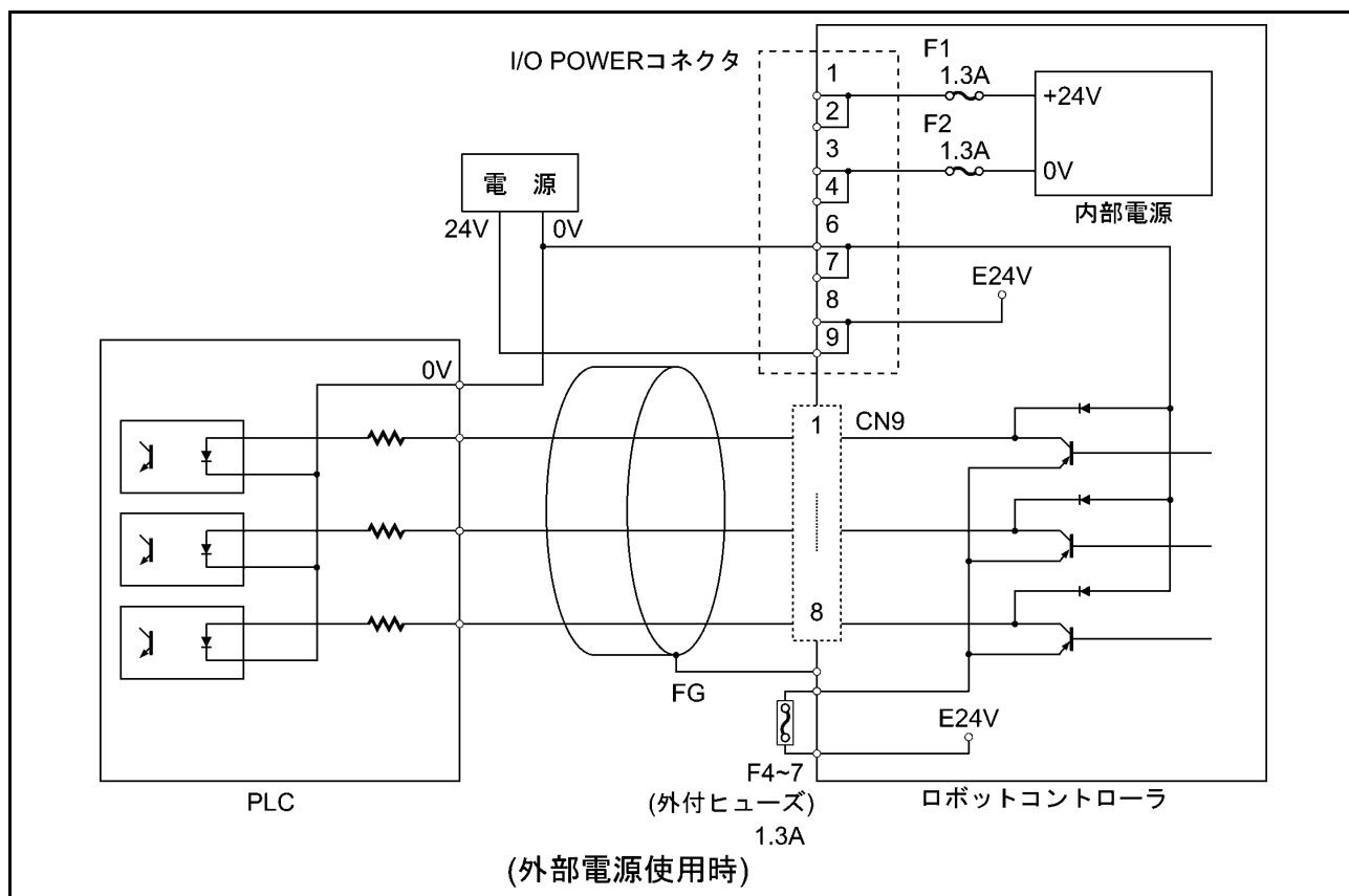
ハンド出力の回路 (PNPタイプI/O)
