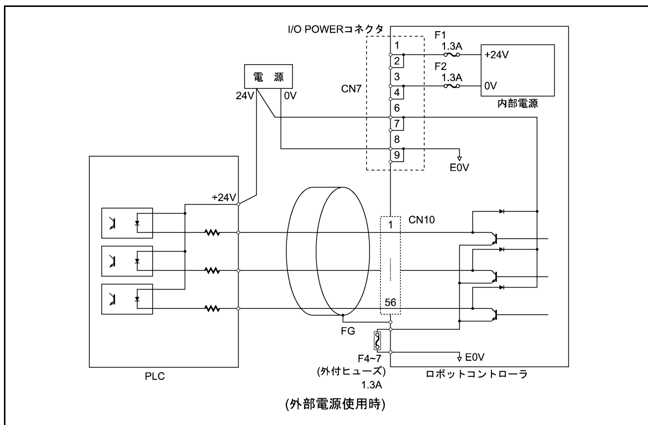
汎用出力・専用出力の回路 (NPNタイプI/O)
