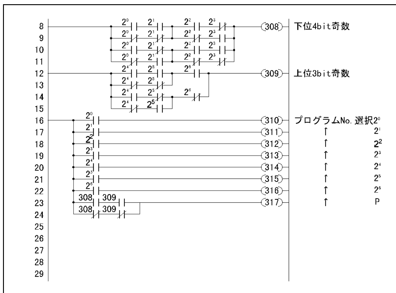
プログラムNo. 選択信号のシーケンス回路例
