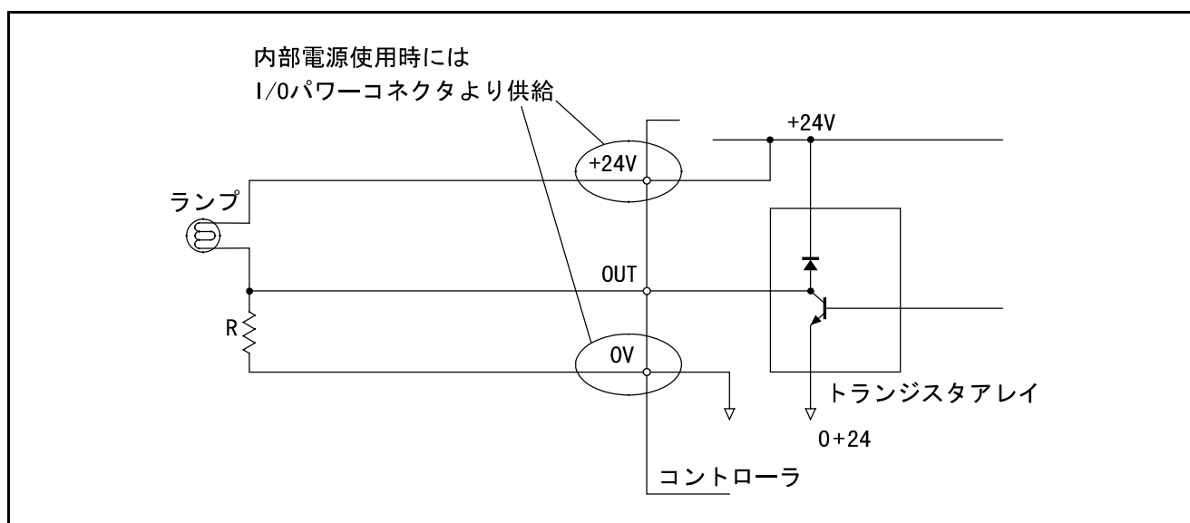
ランプ接続回路例 (NPNタイプI/O)
