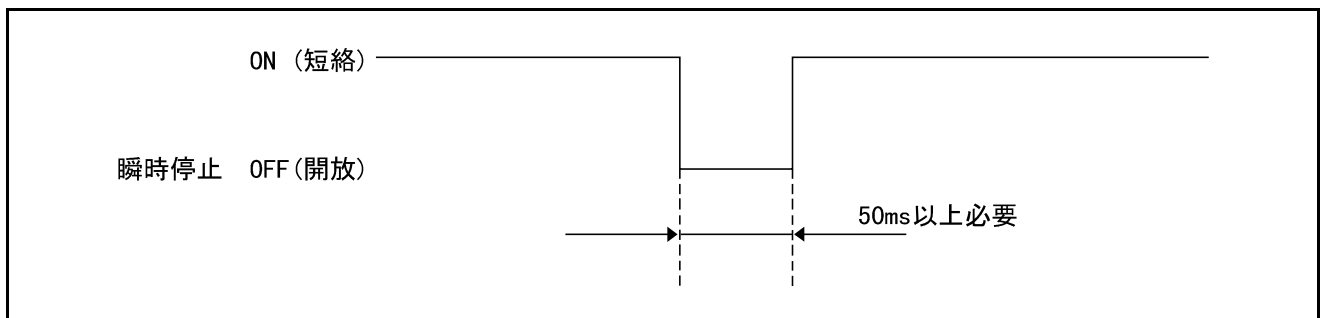
瞬時停止最低パルス幅
