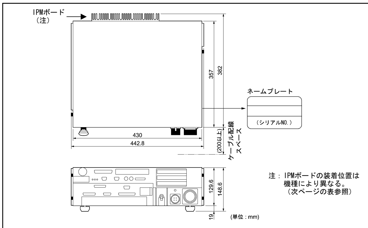
ロボットコントローラの外形寸法 [VM-D/HM-Eシリーズおよび付加軸仕様ロボット用以外]
