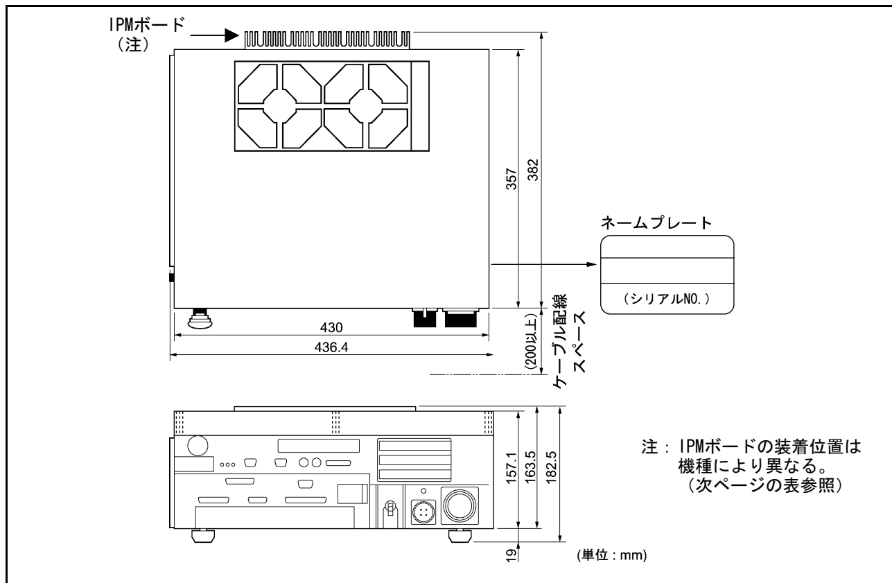
ロボットコントローラの外形寸法 [VM-D/HM-Eシリーズおよび付加軸仕様ロボット用]
