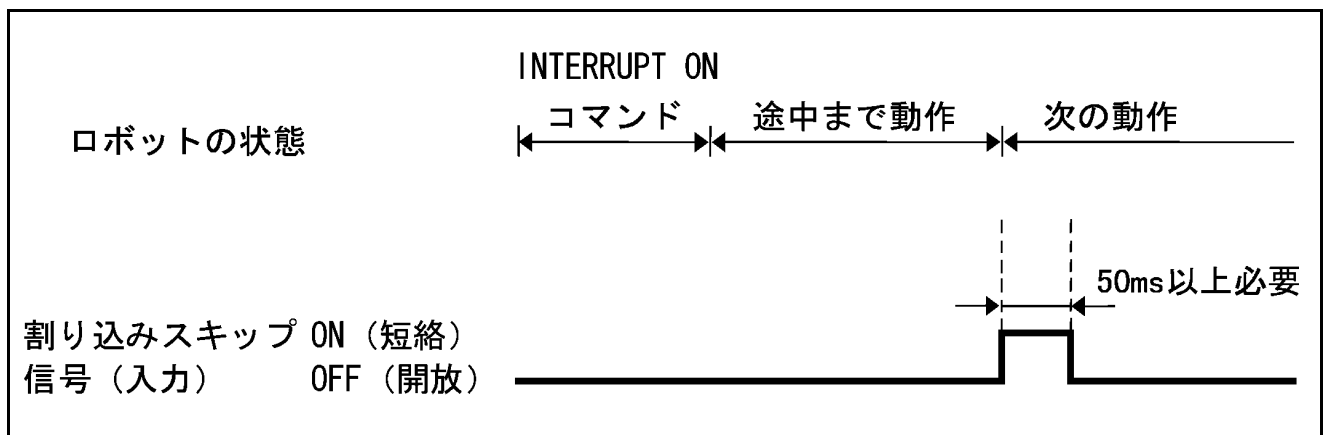
割り込みスキップの入力条件と動作（標準モード）
