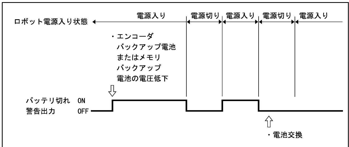
バッテリー切れ警告出力（標準モード）
