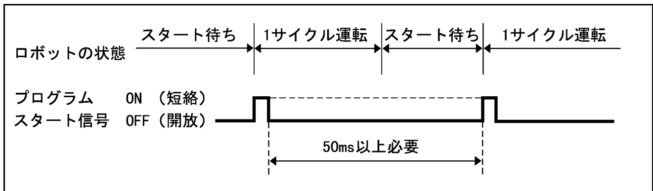
プログラムスタートの動作 1（互換モード）
