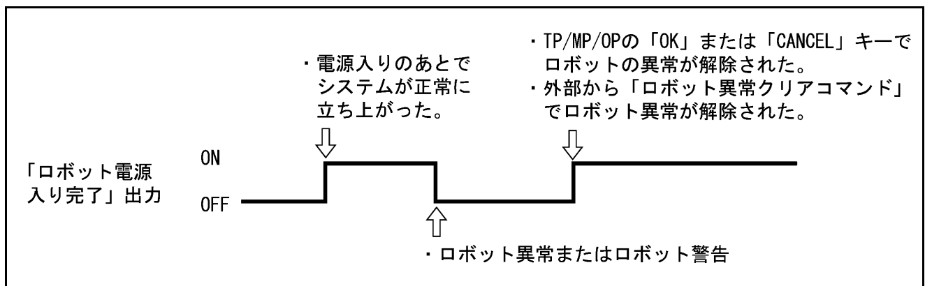
ロボット電源入り完了出力（標準モード）
