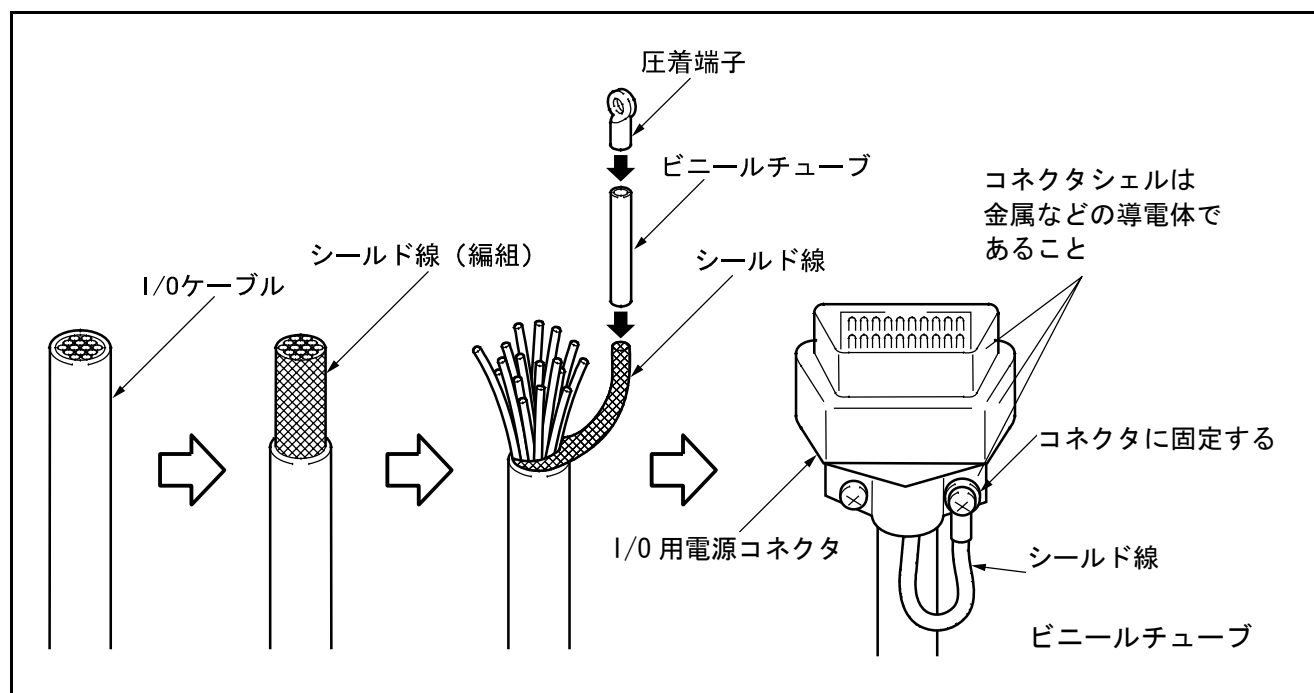
シールド線の処理例
