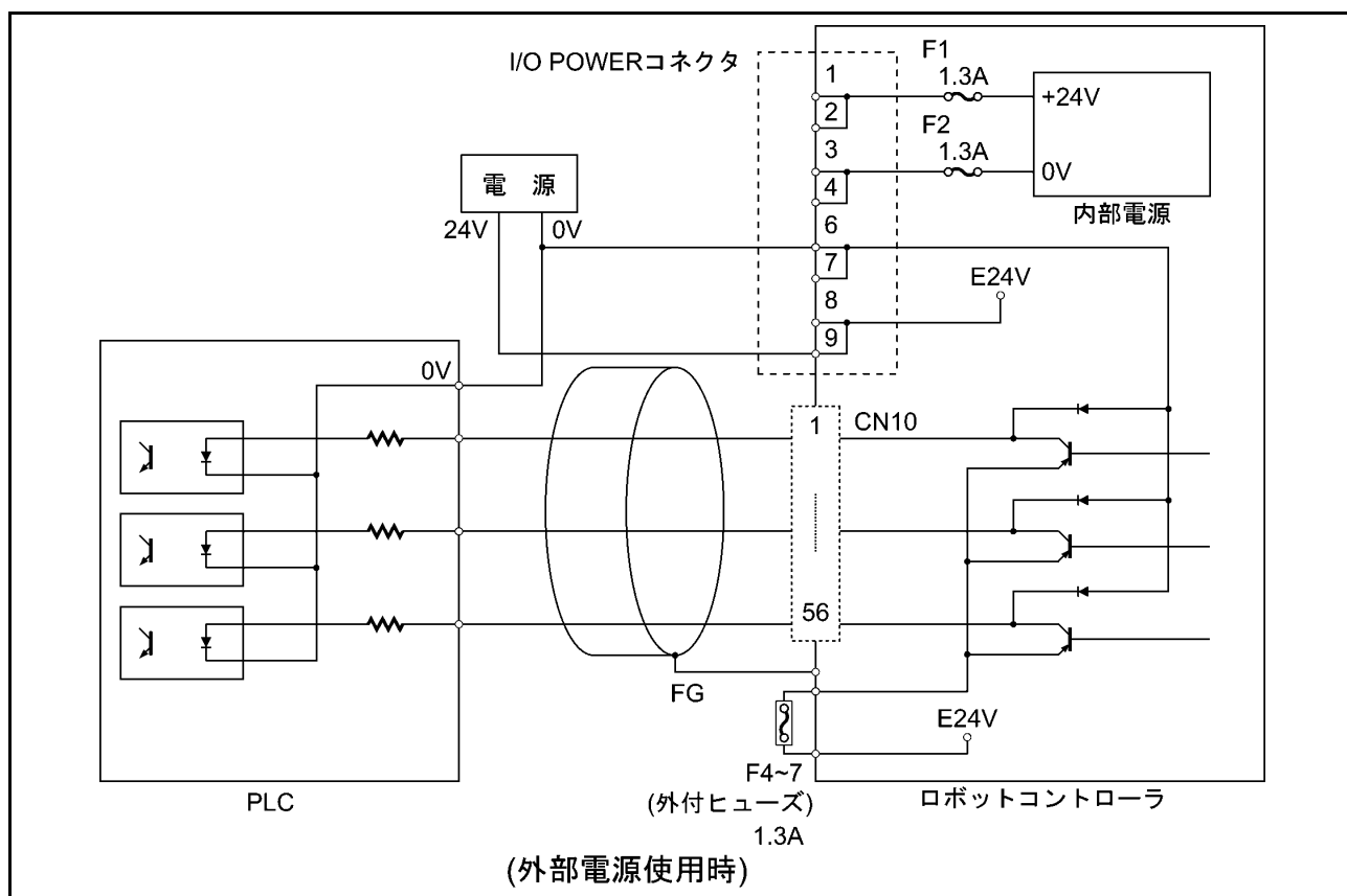
汎用出力・専用出力の回路（PNPタイプI/O）
