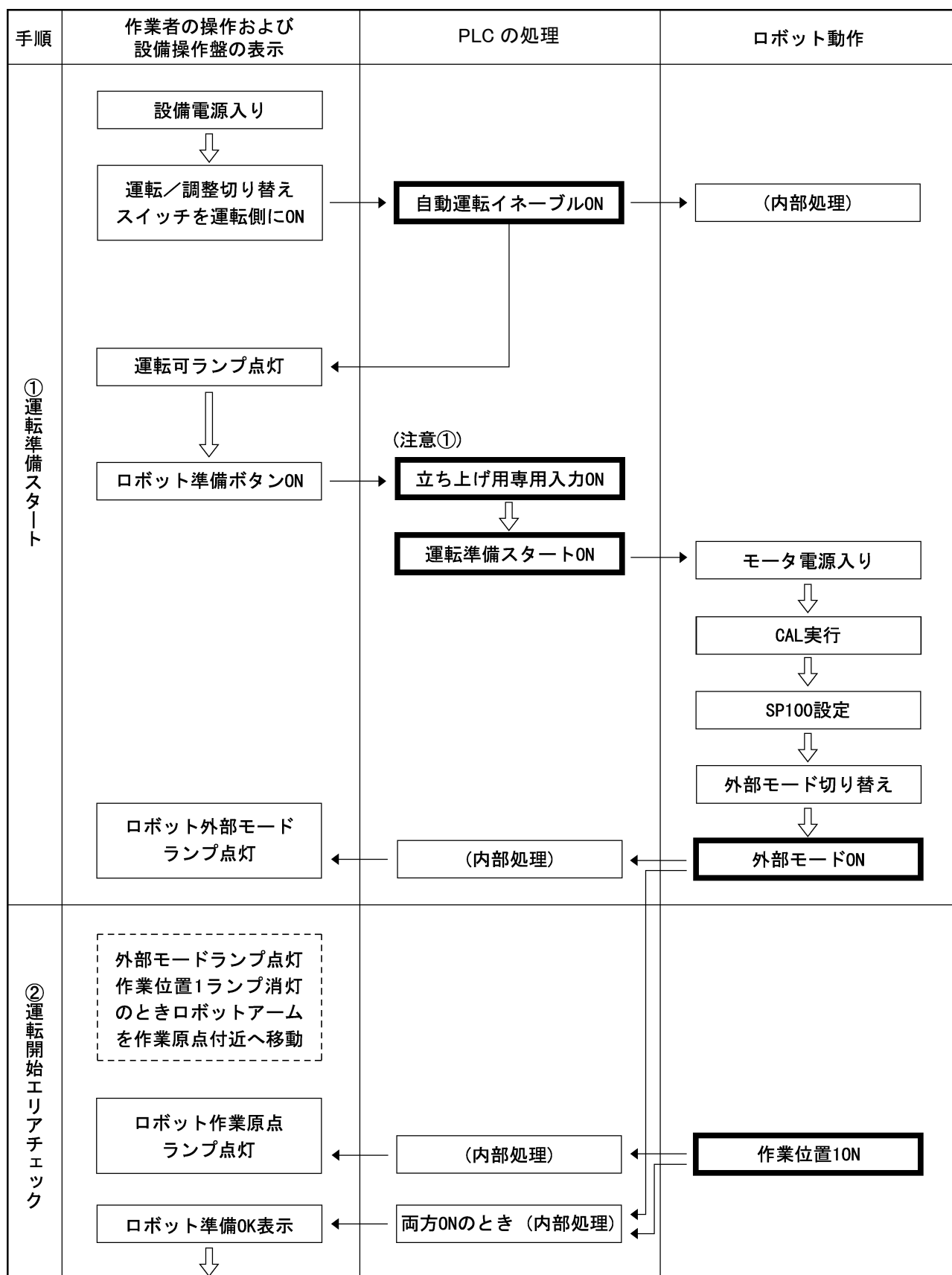
起動・停止の手順と専用入出力信号-1
