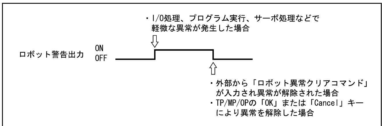
ロボット警告出力（標準モード）
