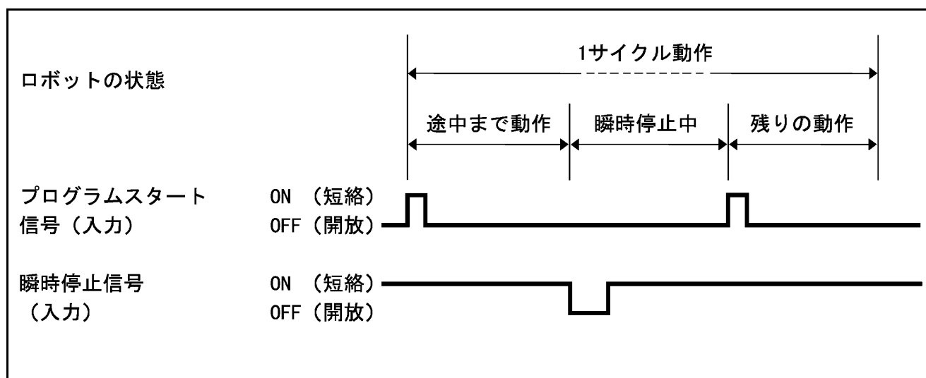
プログラムスタートの動作 3 (互換モード)
