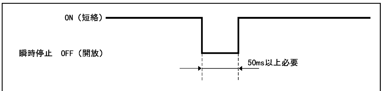
瞬時停止最低パルス幅（標準モード）
