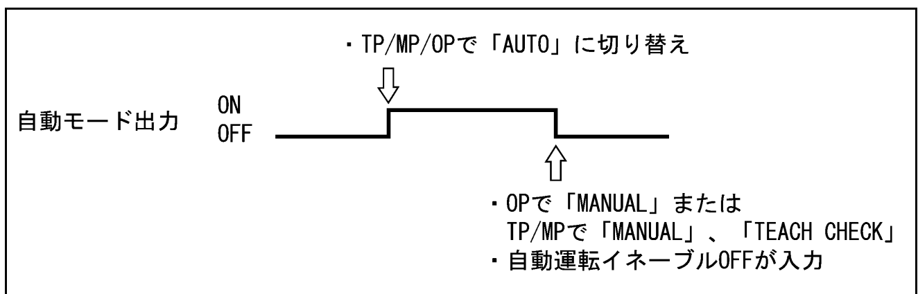
自動モード出力（標準モード）
