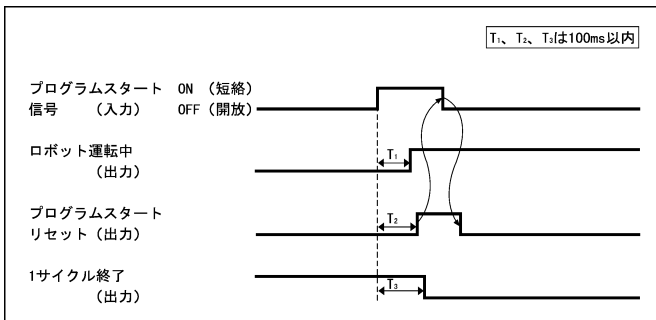
プログラムスタート信号立ち上げの出力信号のタイミング（互換モード）
