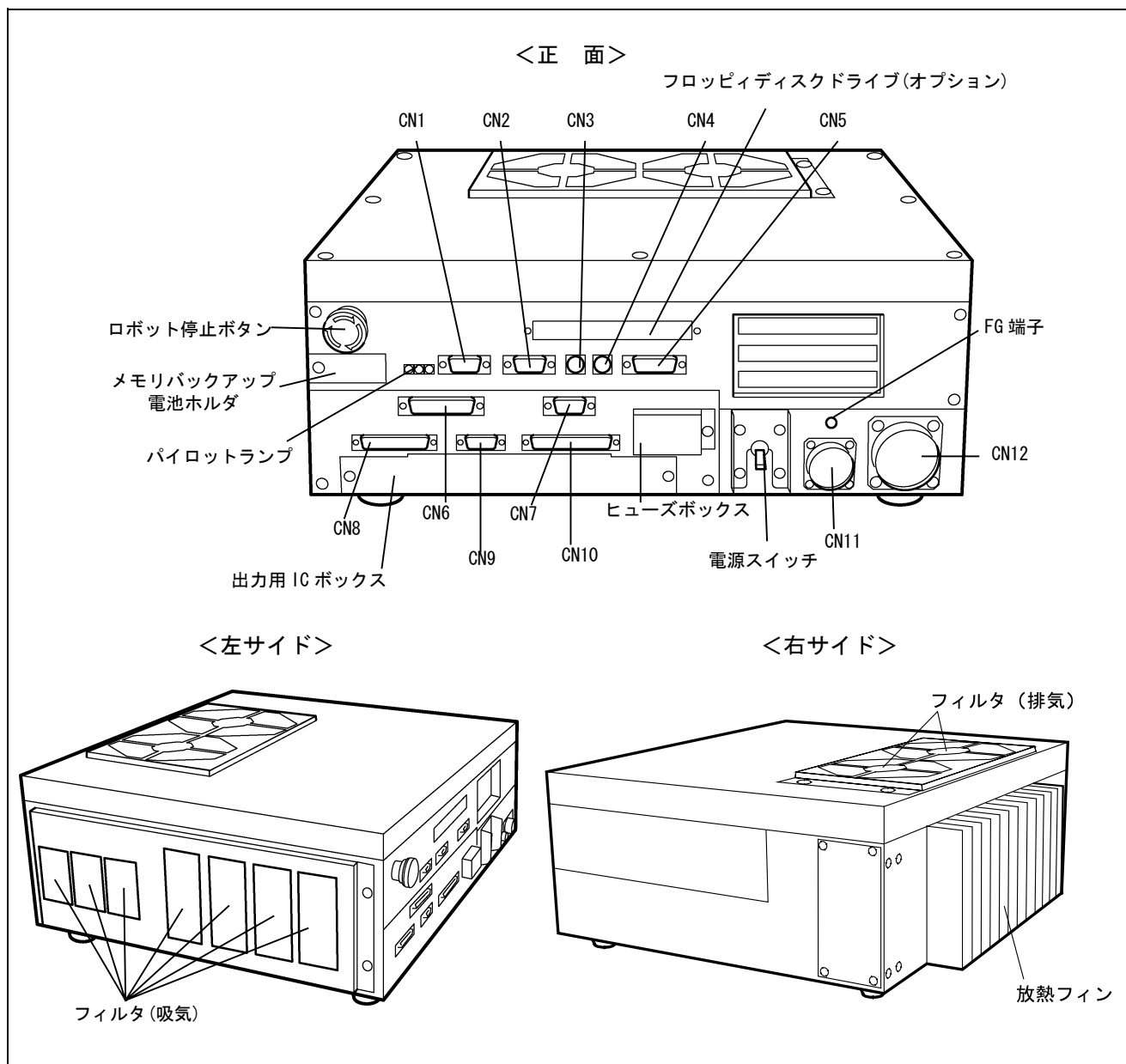
ロボットコントローラ各部の名称 (VM-D/HM-Eシリーズ)
