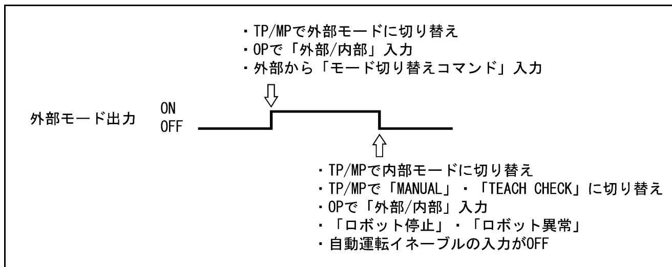
外部モード出力（標準モード）
