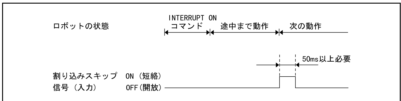
割り込みスキップの入力条件と動作
