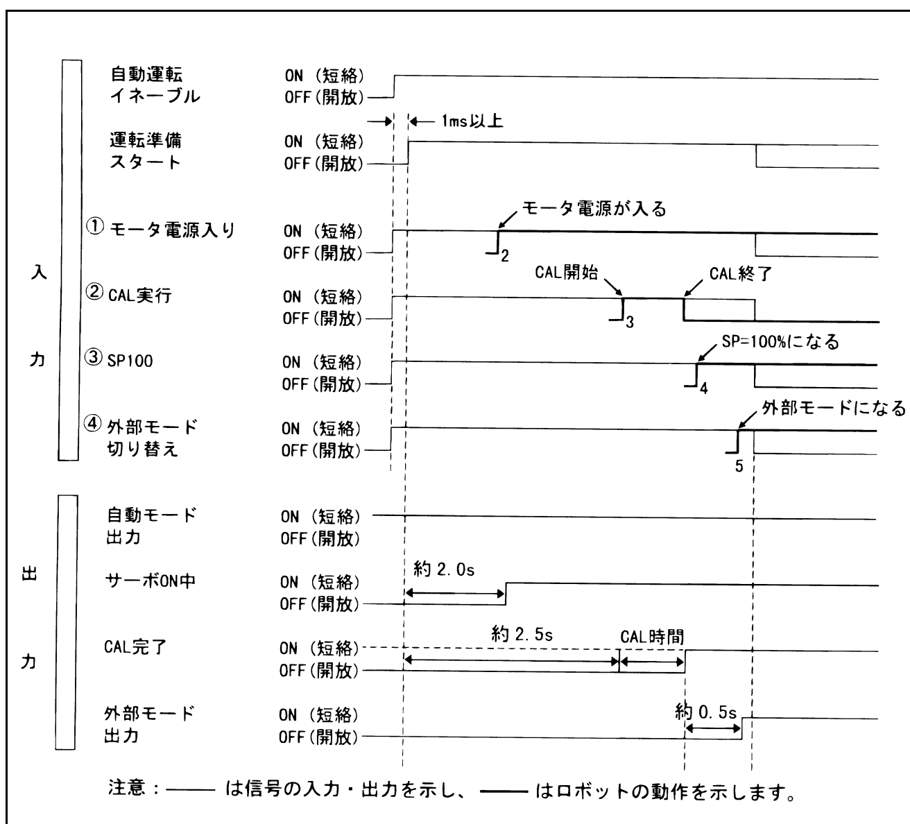
運転準備スタート信号のタイミングチャート例（互換モード）
