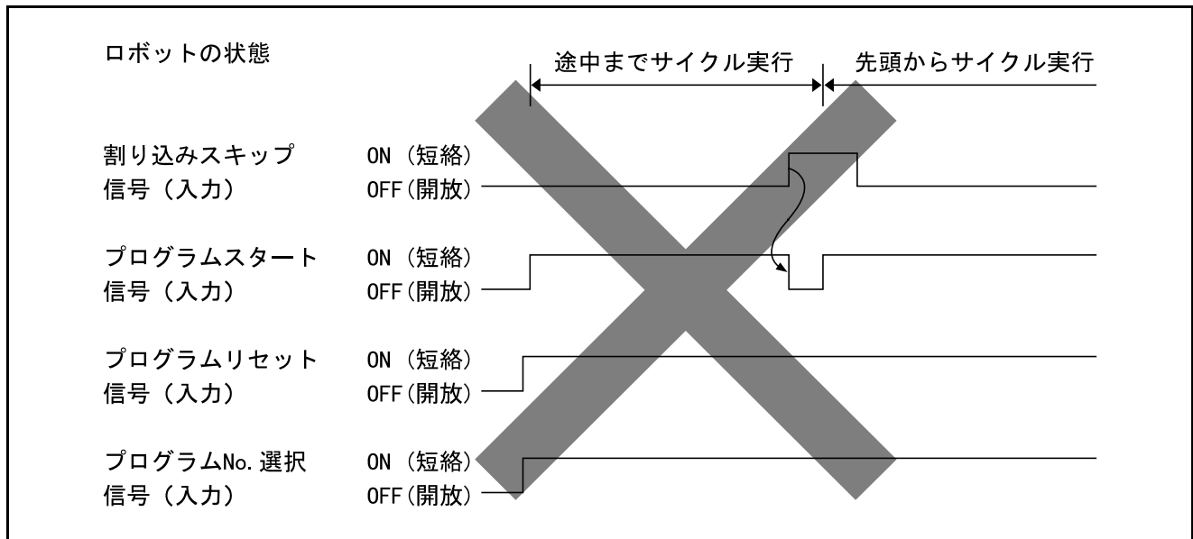
割り込みスキップ入力時の動作例
