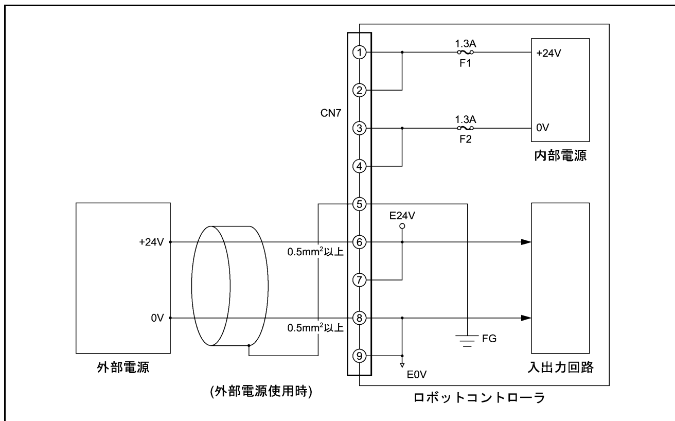
I/Oパワーコネクタ接続例 (NPNタイプI/O)
