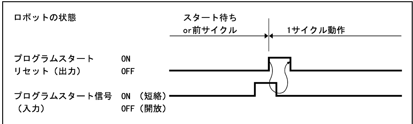
プログラムスタート信号立ち下げのタイミング例 1（互換モード）
