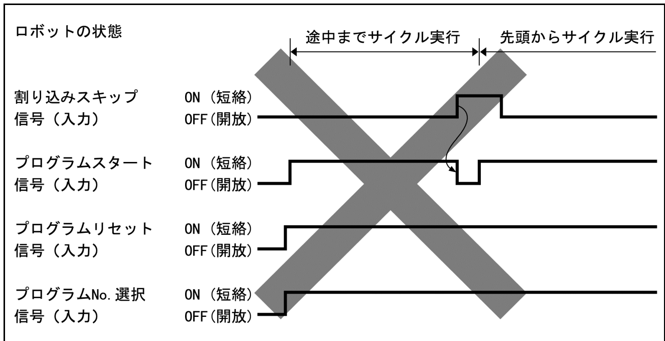
割り込みスキップ入力時の動作例（標準モード）
