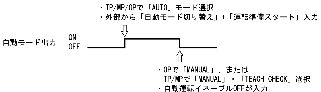
自動モード出力（互換モード）
