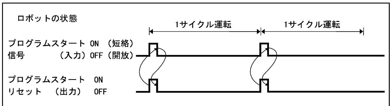
プログラムスタートリセット出力（互換モード）
