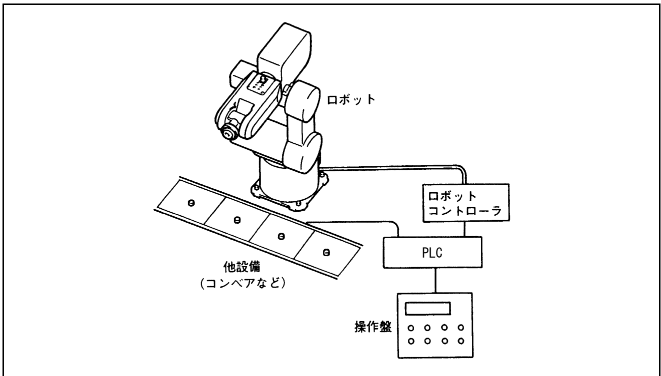
ロボットを使った設備例（標準モード）
