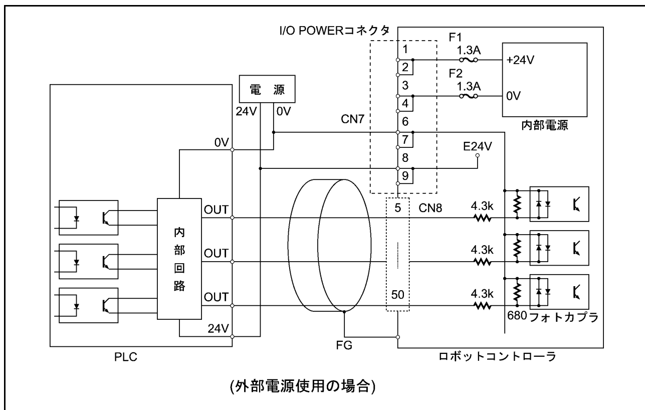
汎用入力・専用入力の回路 (PNPタイプI/O)
