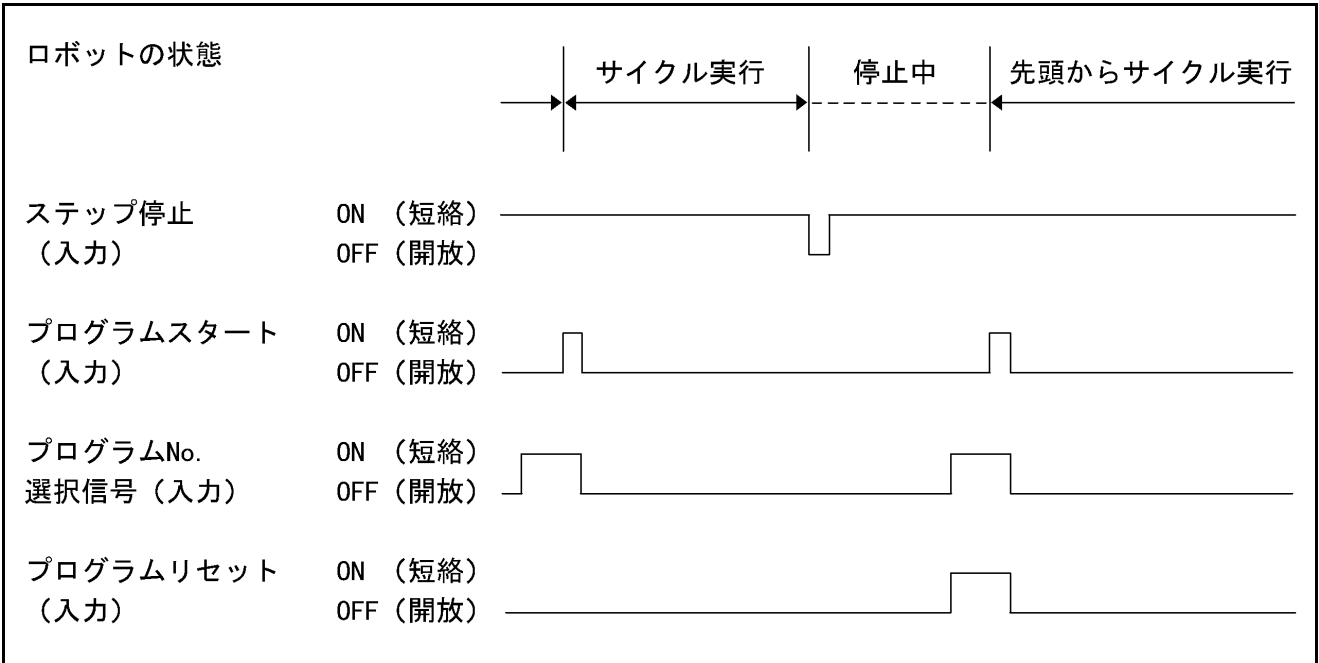
プログラムのリセット信号の入力条件と動作
