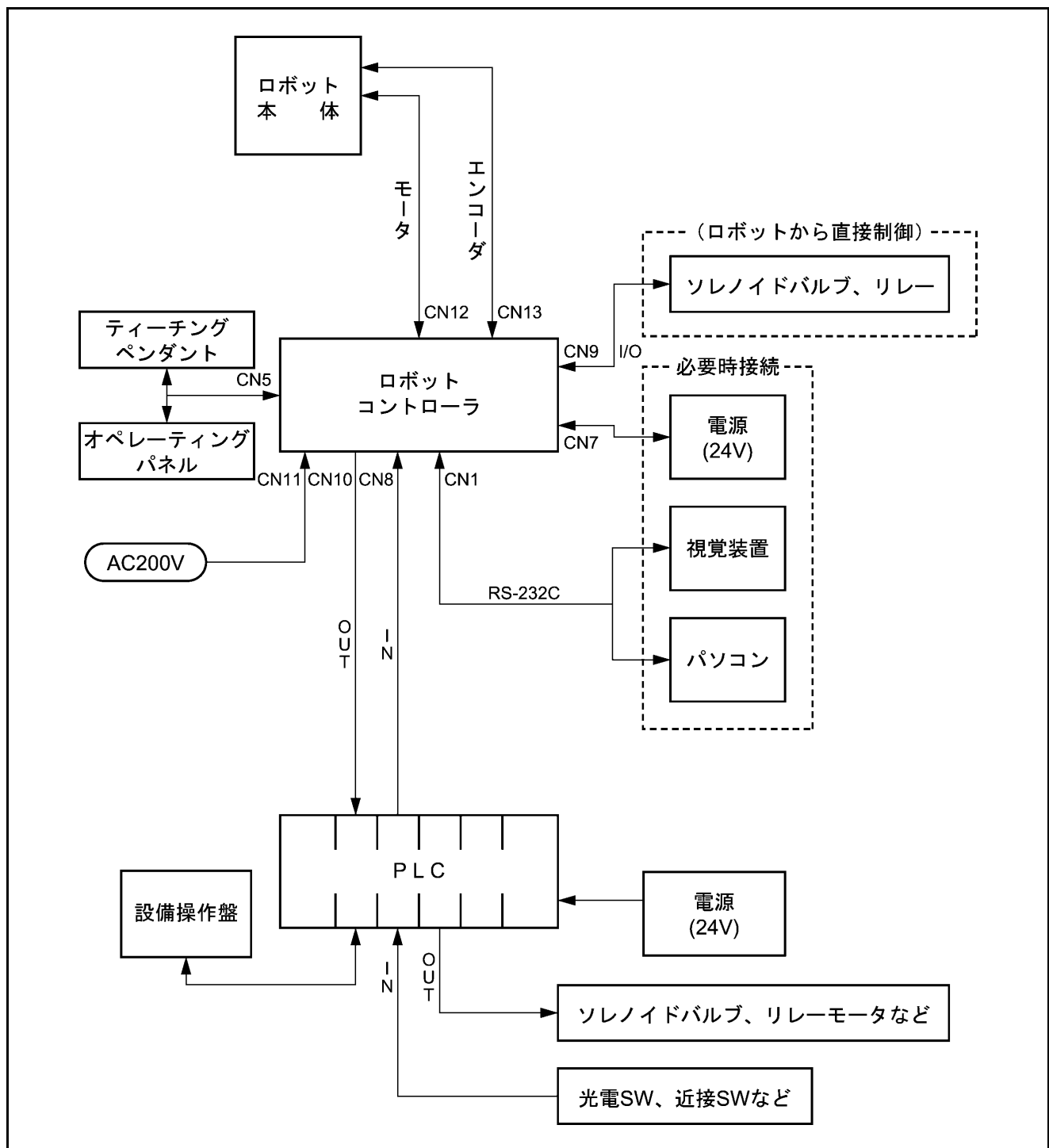
システムの構成例
