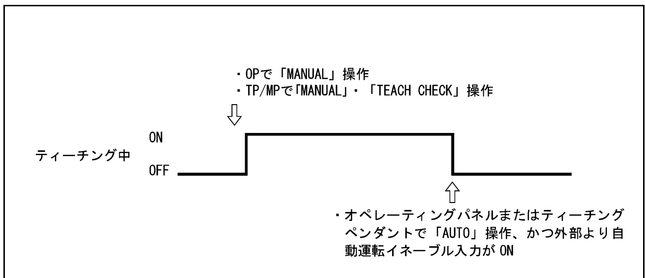
ティーチング中出力（互換モード）
