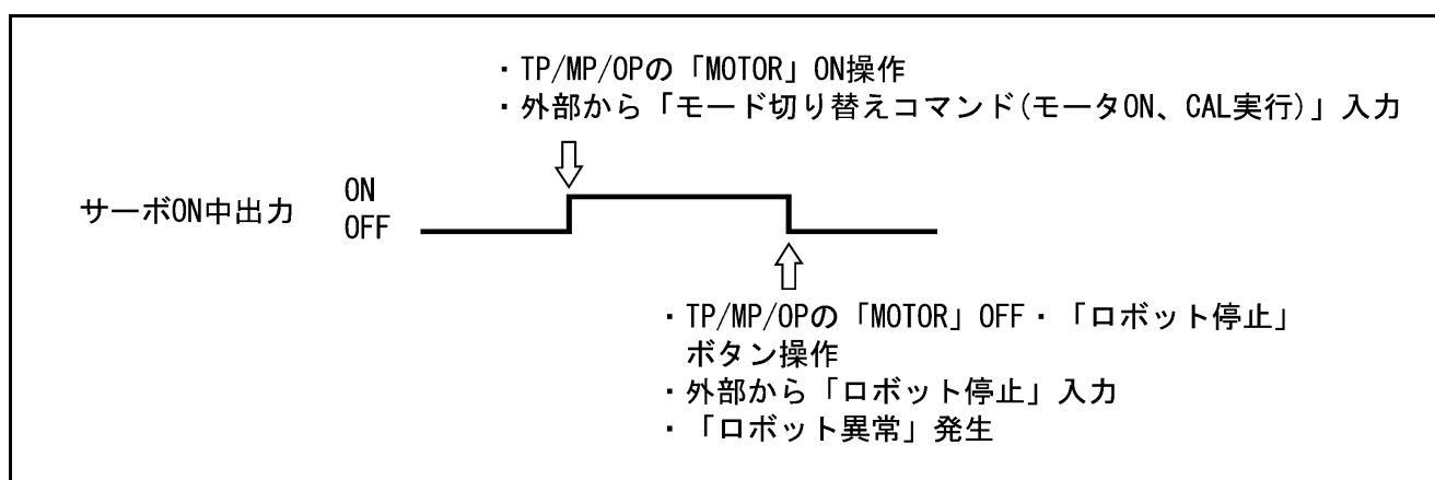
サーボON中出力（標準モード）
