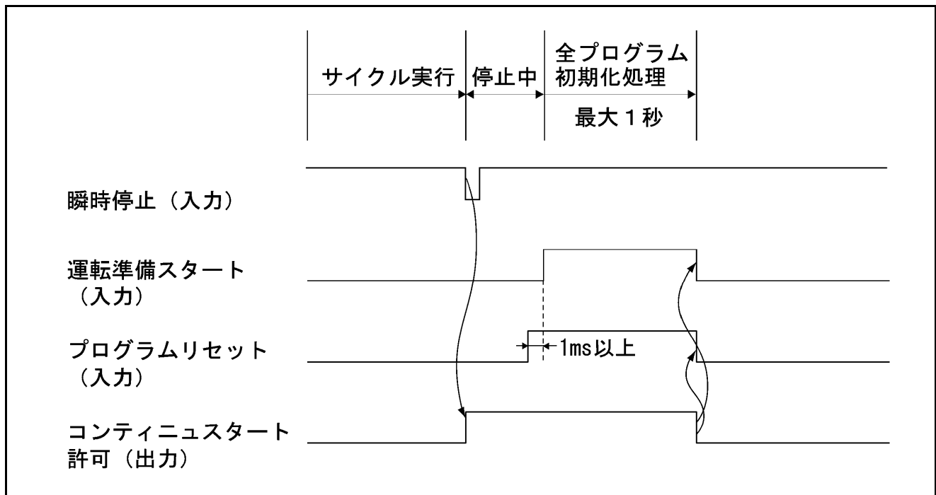
プログラムリセット信号の入力条件と動作
