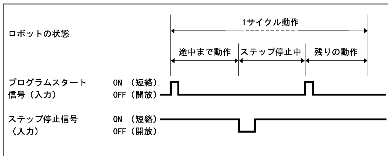
プログラムスタートの動作 2 (互換モード)
