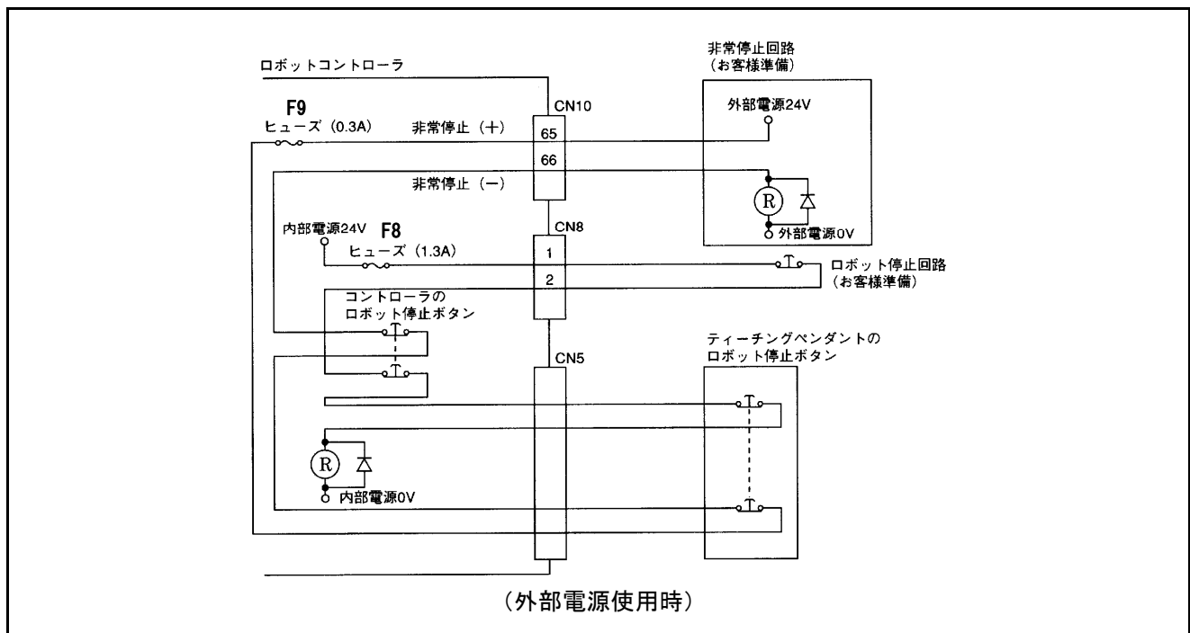
非常停止回路（標準仕様）
