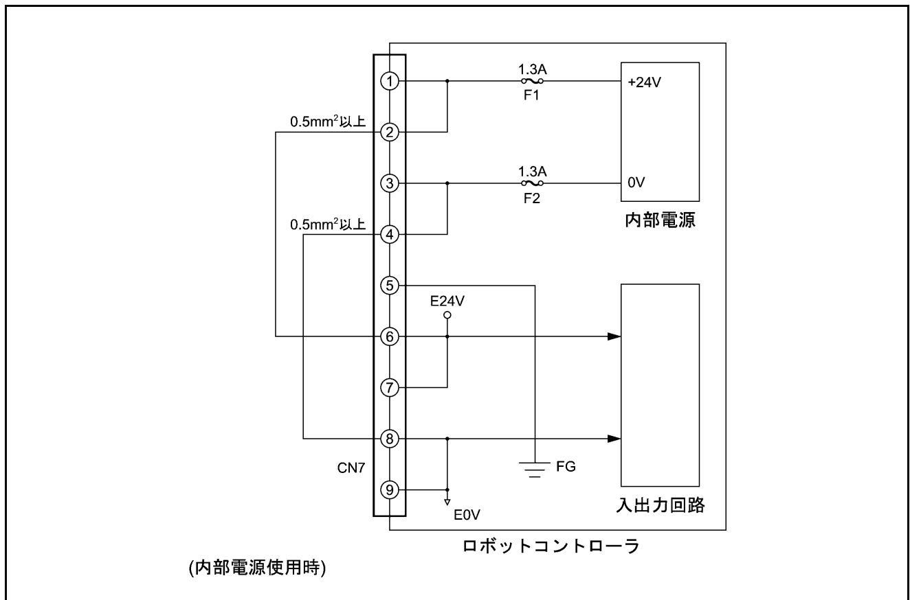
I/Oパワーコネクタ接続例 (NPNタイプI/O)
