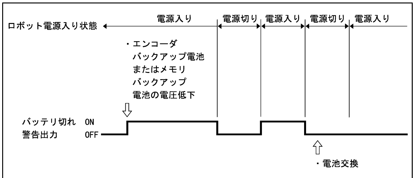
バッテリー切れ警告出力（互換モード）
