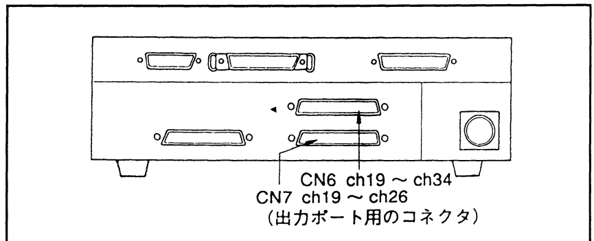
図 8-48 出力ポートのコネクタ位置
