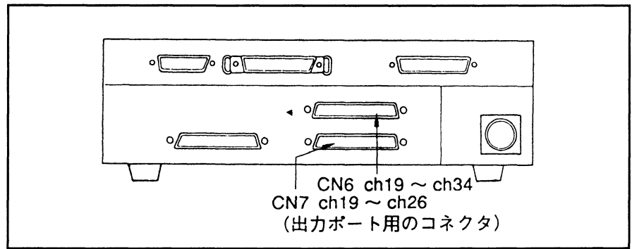
図 8-50 出力ポートのコネクタ位置
