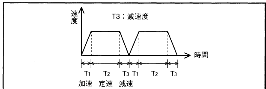
図8-26 減速度
