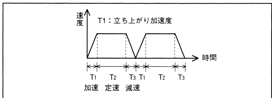
図8-25 立ち上がり加速度
