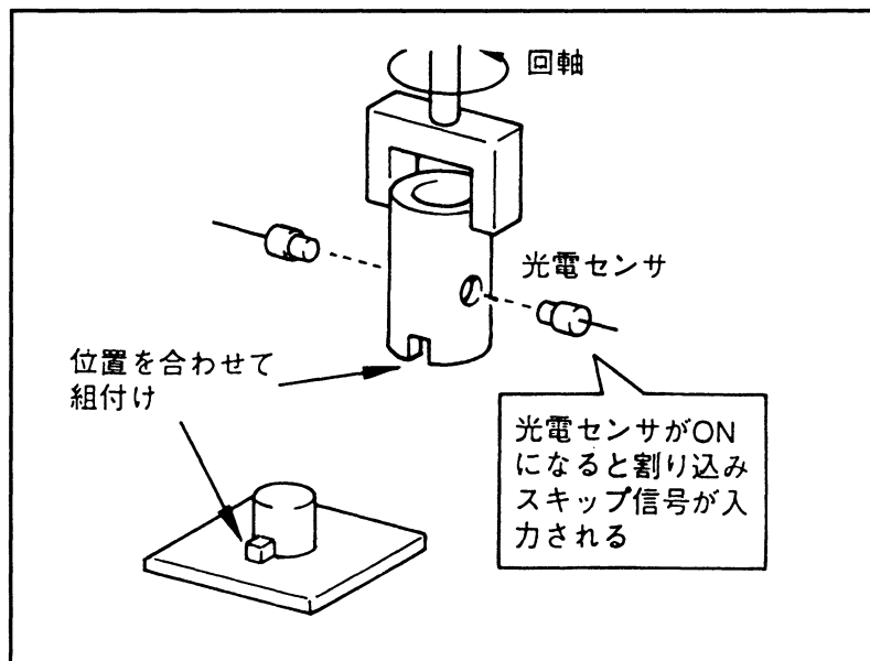
図8-44 INTRPTコマンドのプログラム例説明図
