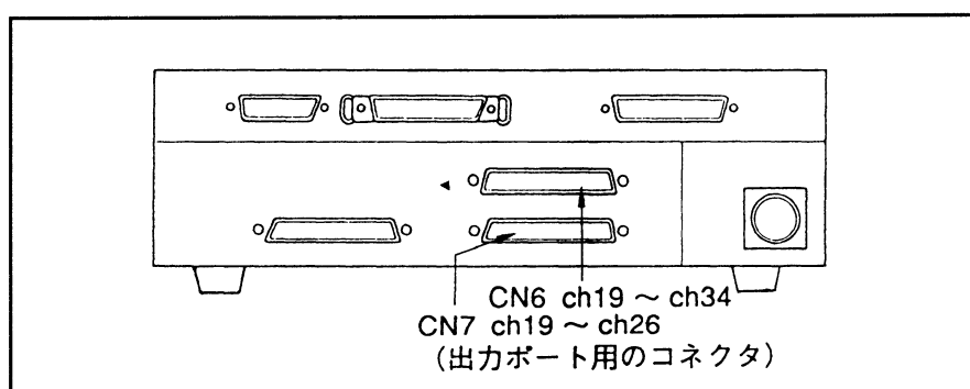
図8-53 出力ポートのコネクタ位置
