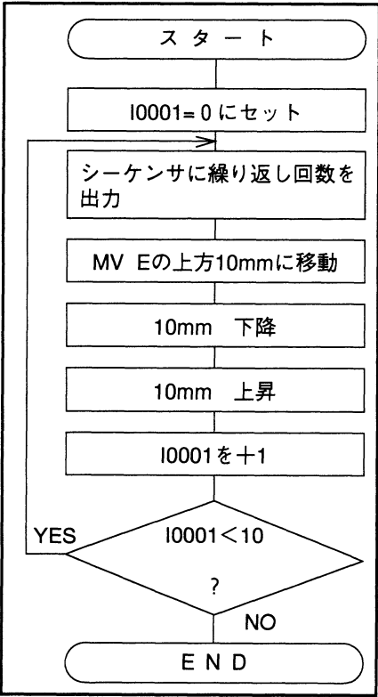
図8-76 プログラム例のフローチャート
