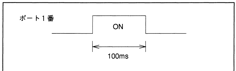
図 8-51 プログラム例 (2) の動作
