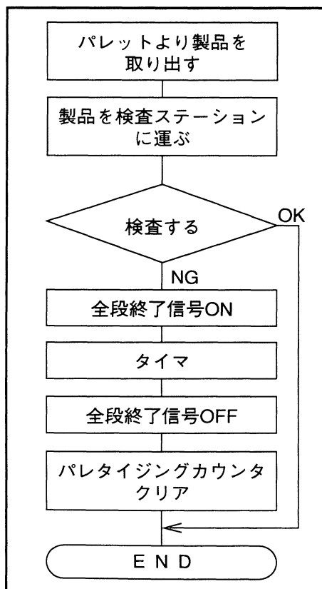
図 8-70 プログラム例のフローチャート
