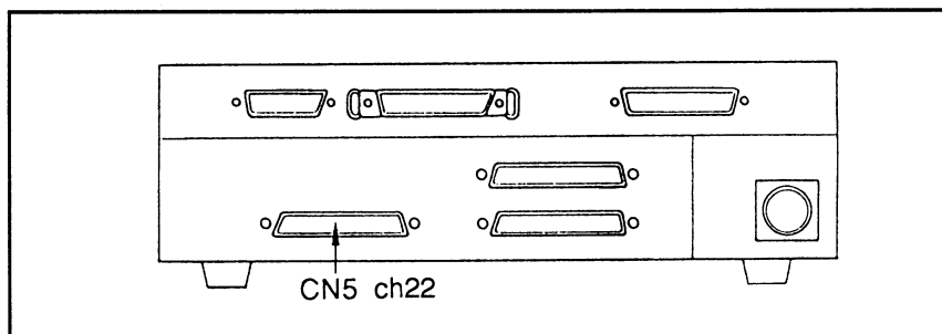
図8-43 割り込みスキップ信号入力用コネクタ位置
