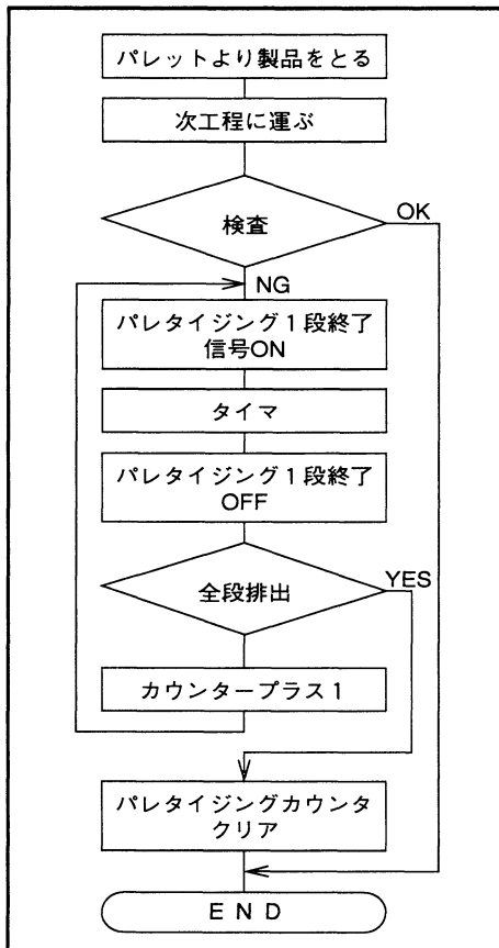
図8-65 プログラム例の フローチャート
