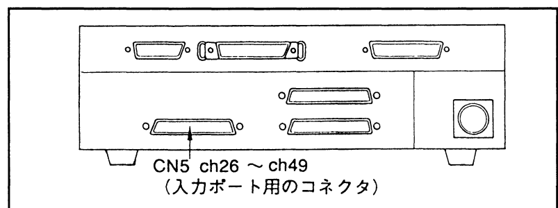
図8-33 入力ポートのコネクタ位置
