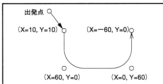
図8-7 DRWコマンドのプログラム例
