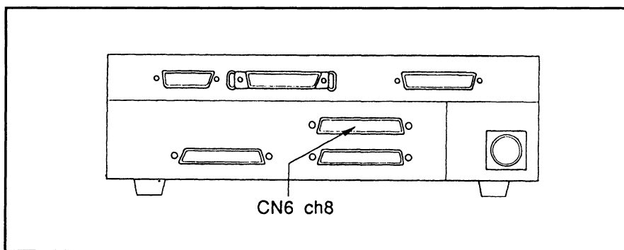
図 8-72 パレタイジグ全段終了信号のコネクタ配置図
