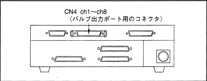
図8-61 バルブ出力ポートのコネクタ位置
