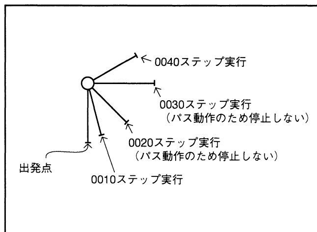
図8-5 プログラム例の動作軌跡
