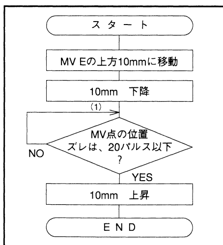
図8-38 プログラム例(1)のフローチャート
