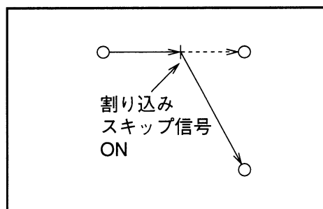
図8-41 割り込みスキップ信号がONされたとき
