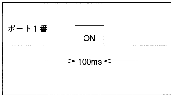
図 8-54 プログラム例 (1) の動作
