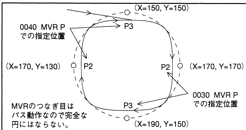
図8-21 プログラム例(3)の動作軌跡
