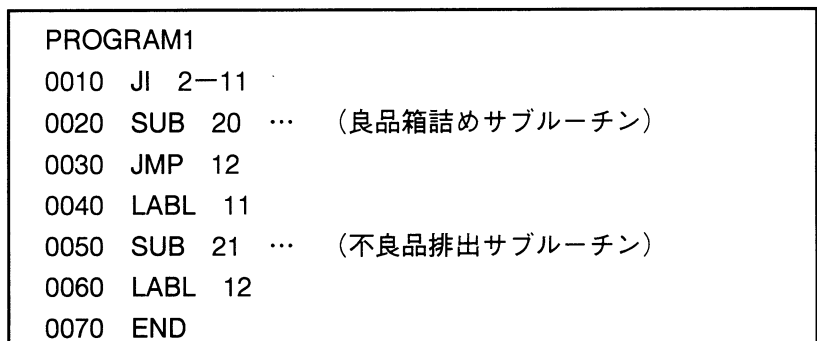
図8-29 JIコマンドのプログラム例
