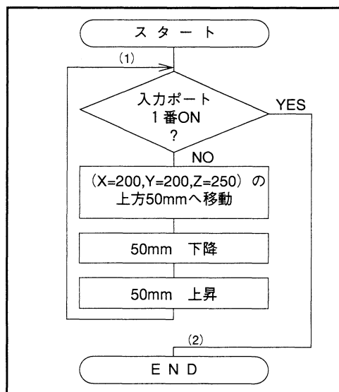
図8-34 プログラム例のフローチャート
