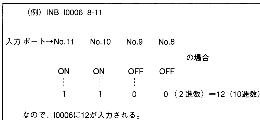
図8-74 数値入力の場合
