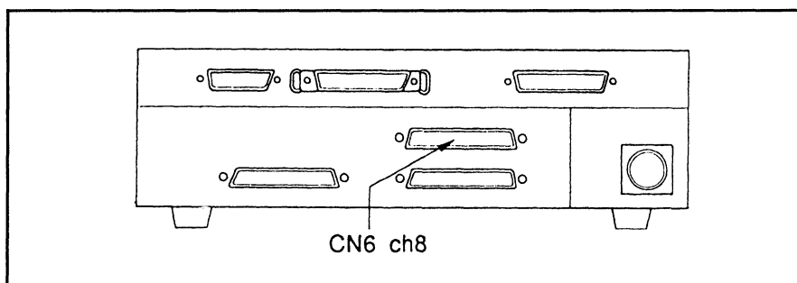
図 8-69 パレタイジング全段終了信号のコネクタ位置
