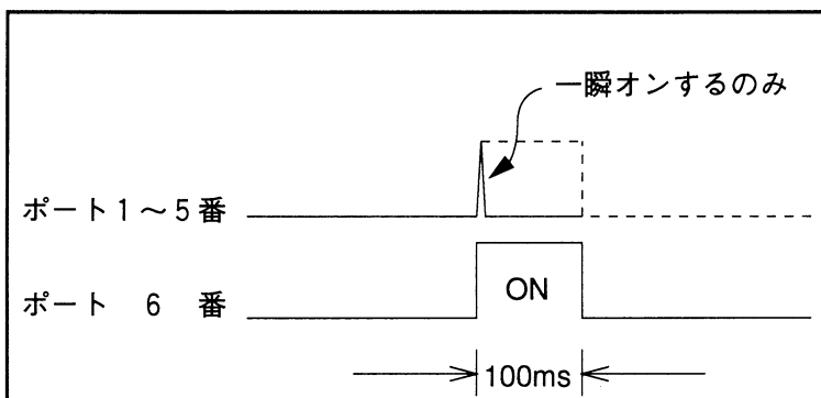
図 8-56 プログラム例 (2) の動作
